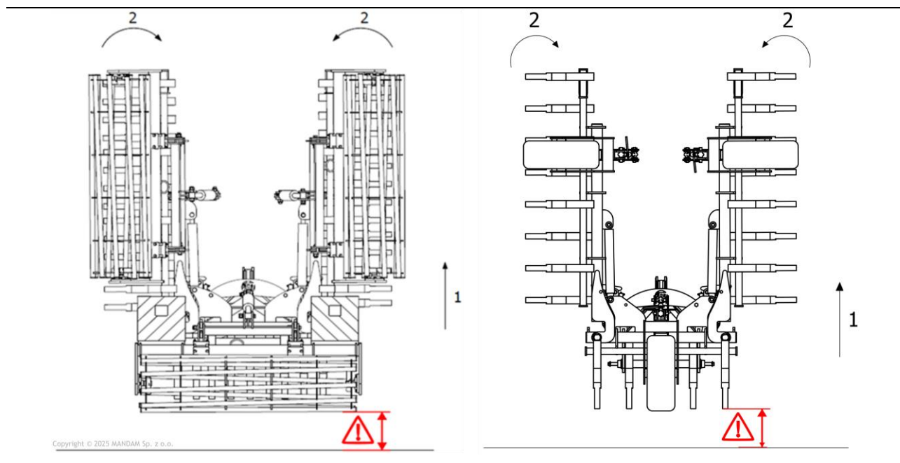
Rysunek 8 Sekwencja otwierania maszyny (1 - podniesienie maksymalnie (co najmniej 60 cm) maszyny w górę, 2 - złożenie skrzydeł maszyny do pozycji „zamkniętej”).
