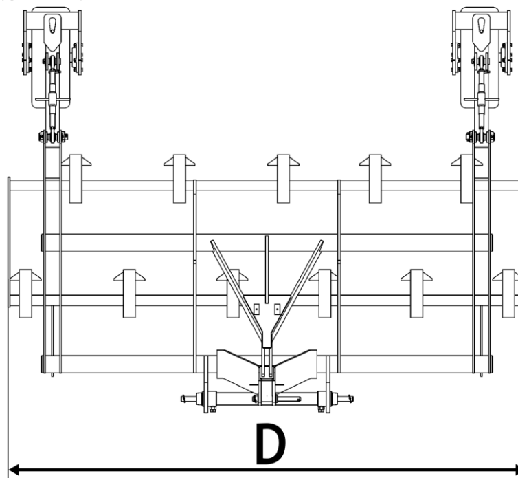
Rysunek 23 Wymiary transportowe kultywatora SUPER FRONT 3,00m (L - długość, H - wysokość, D - szerokość) (patrz tabela 4)
