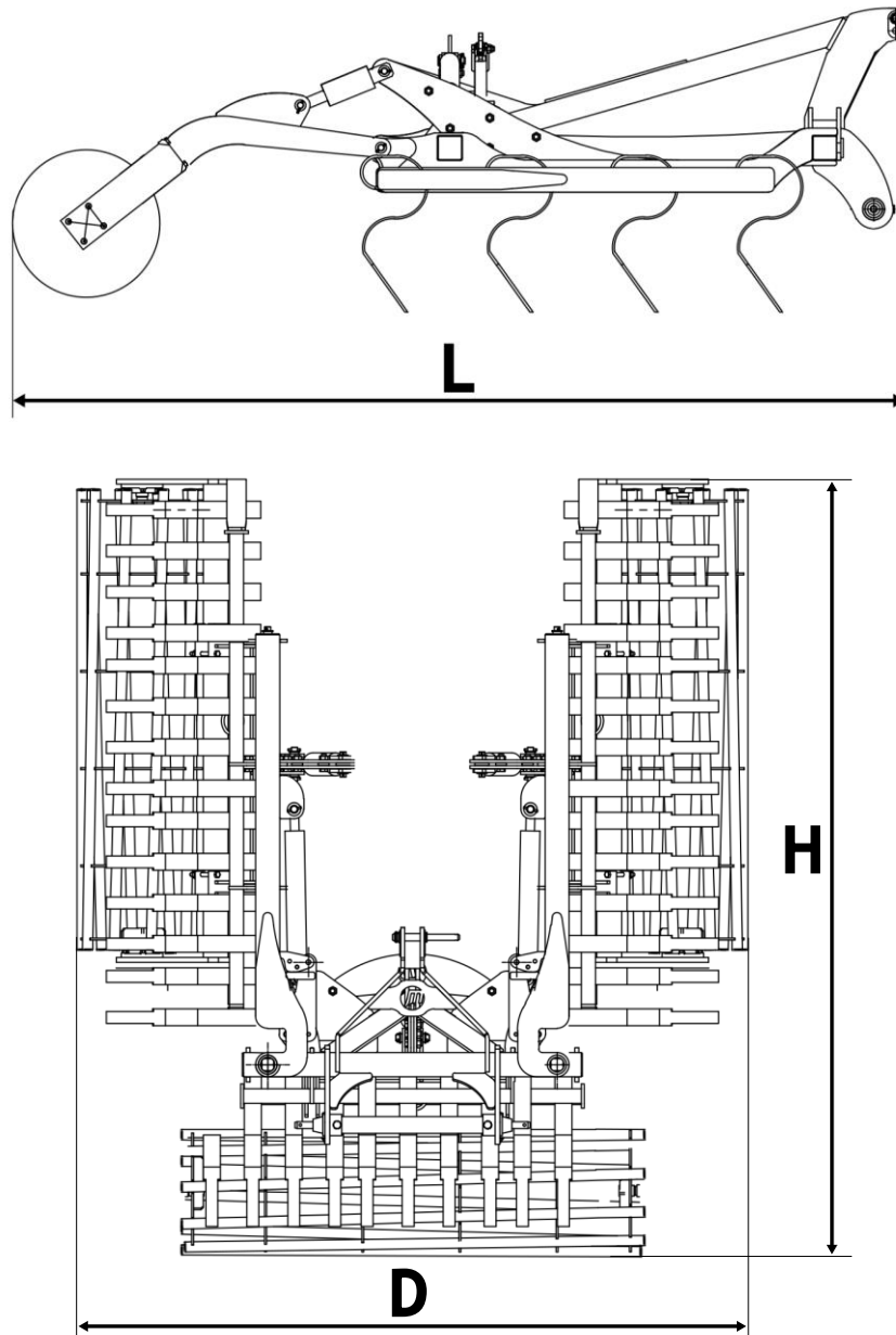
Rysunek 22 Wymiary transportowe kultywatora SUPER o szerokościach 4.00m, 5.00m oraz 6.00m z opcją wału rurowego (L - długość, H - wysokość, D - szerokość)(patrz tabela 3)
