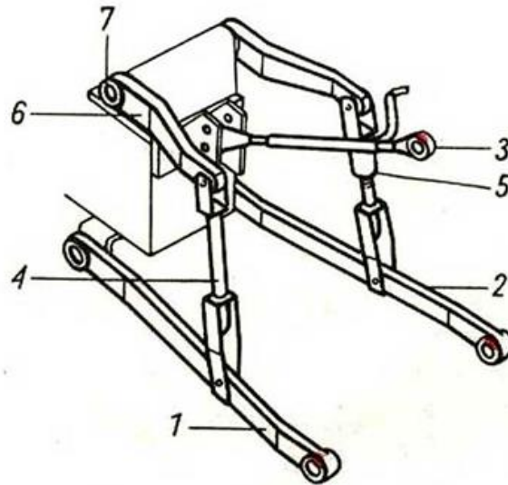
Rysunek 6 Trzypunktowy układ zawieszenia TUZ ciągnika: 1,2 - cięgna dolne, 3 - łącznik górny, 4 - wieszak lewy, 5 - wieszak prawy o regulowanej długości, 6 - ramię podnośnika, 7 - wał podnośnika
