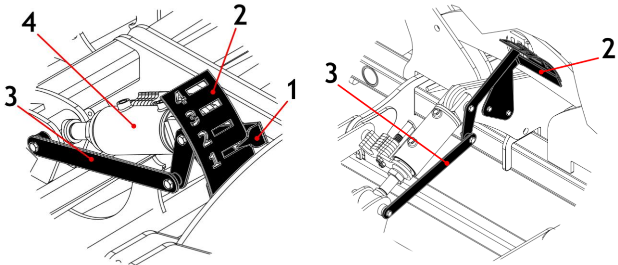
Widok z boku (punkty montażu wskaźnika)
