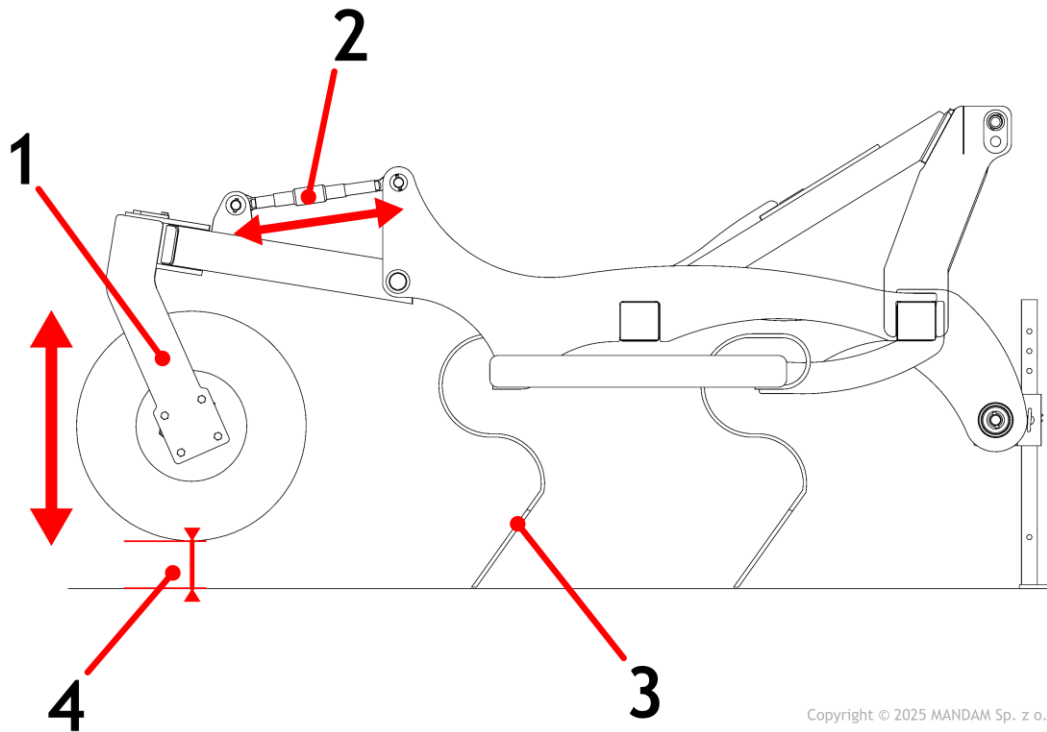
Rysunek 16 Regulacja głębokości pracy (1 - koło podporowe, 2 - śruba rzymska, 3 - ząb sprężynowy, 4 - głębokość robocza)
