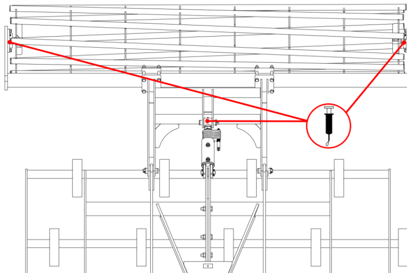
Rysunek 18 Punkty smarowania kultywatora SUPER w wersji nieskładanej hydraulicznie (opcja z wałem rurowym)
