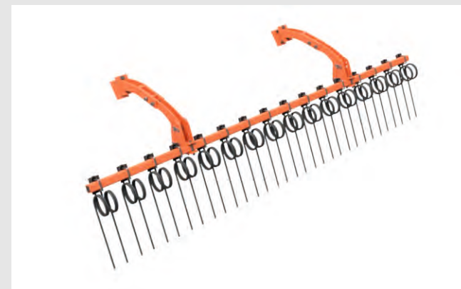
BELKA Z PAŻURKAMI ZA WAŁEM
