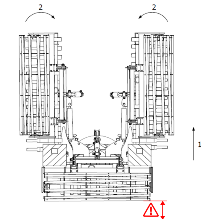
Rysunek 8 Sekwencja otwierania maszyny (1 - podniesienie maksymalnie (co najmniej 60 cm) maszyny w górę, 2 - złożenie skrzydeł maszyny do pozycji „zamkniętej”).
