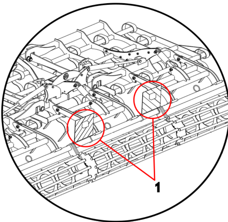
Rysunek 15 Tablice oświetleniowe oraz ich umiejscowienie. (na przykładzie kultywatora składanego hydraulicznie) (1 - tablice oświetleniowe)
