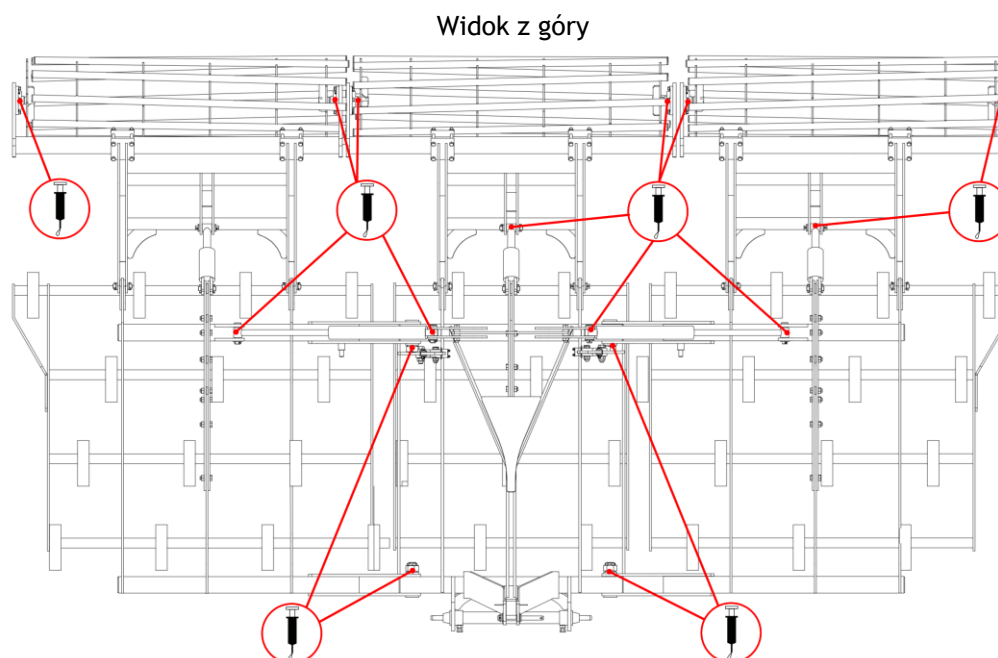
Rysunek 17 Punkty smarowania kultywatora SUPER w wersji składanej hydraulicznie (opcja z wałem rurowym)
