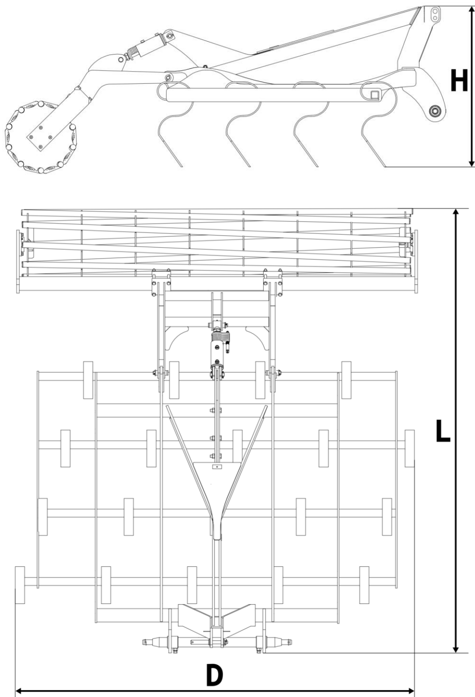
Rysunek 18 Gabaryty transportowe kultywatora SUPER o szerokości 3,00m z opcją wału rurowego (L - długość, H - wysokość, D - szerokość)
