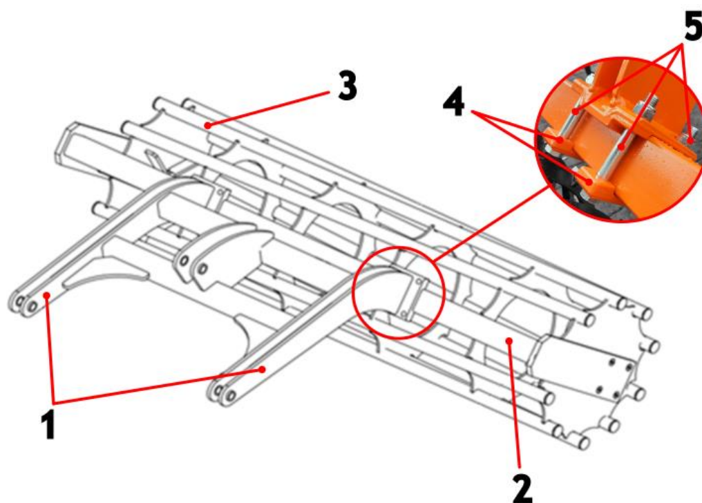
Rysunek 5 Budowa zespołu ramion z wałem rurowym (1 - ramiona wału, 2 - obejma wału rurowego, 3 - wał rurowy (opcja), 4 - płytki mocujące, 5 - śruby mocujące)
