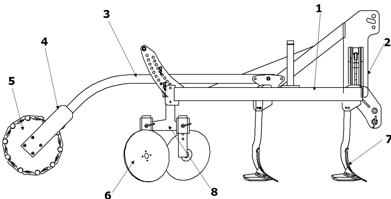
Rys. 1 Budowa kultywatora KUS B: 1 - rama kultywatora, 2 - wieża trójpunktowego układu zawieszenia, 3 - ramie wału, 4 - obejma wału, 5 - wał, 6 - talerz wyrównujący, 7 - grządziel, 8 - uchwyt talerzy wyrównujących.
