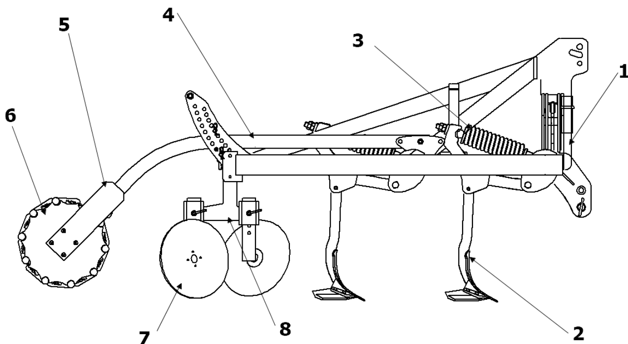
Rys. 2 Budowa kultywatora KUS S: 1 - rama z trójpunktowym układem zawieszenia, 2 - grządziel, 3 - układ sprężynowy, 4 - ramię wału, 5 - obejma wału, 6 - wał, 7 - talerz wyrównujący, 8 - uchwyt talerzy wyrównujących.
