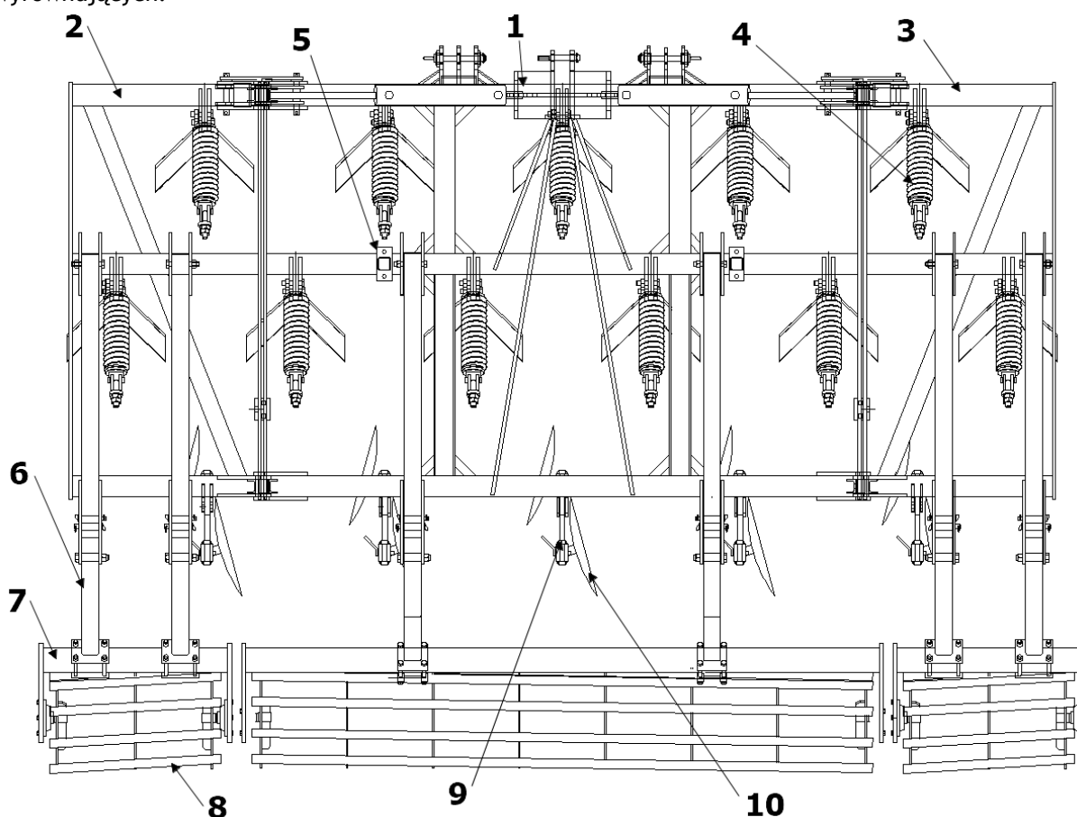
Rys. 3 Budowa kultywatora KUS 3.8, KUS 4.8, KUS 5.6: 1 - rama środkowa z trójpunktowym układem zawieszenia, 2 - rama lewa, 3 - rama prawa, 4 - układ sprężynowy z grządzielem, 5 - wspornik ram bocznych, 6 - ramię wału, 7 - obejma wału, 8 - wał, 9 - uchwyt talerzy wyrównujących, 10 - talerz wyrównujący.
