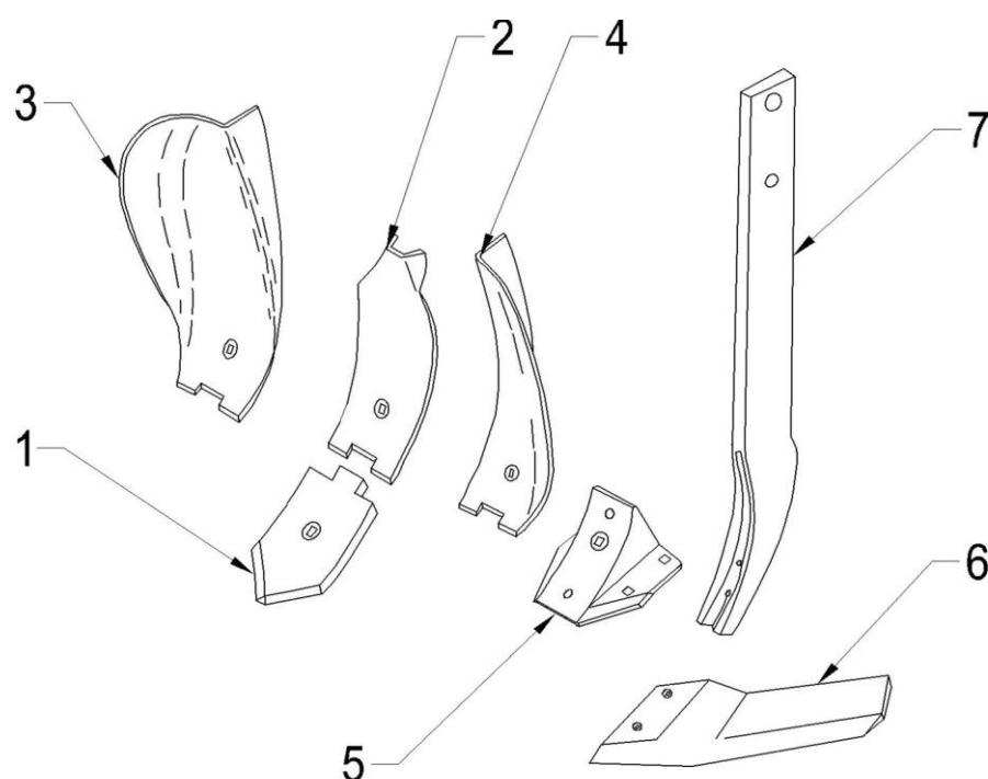
Rys. 4 Budowa elementu roboczego kultywatora KUS: 1 - szpic, 2 - odkładnica środkowa, 3 - odkładnica prawa, 4 - odkładnica lewa, 5 - stopa lemiesza, 6 - lemiesz lewy/prawy, 7 - grządziel.
