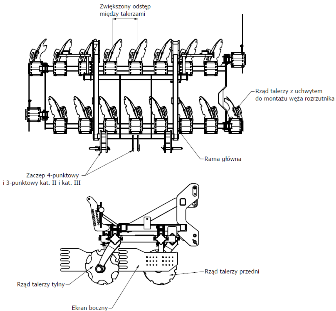
Rys.1 Brona talerzowa GAL-M.
