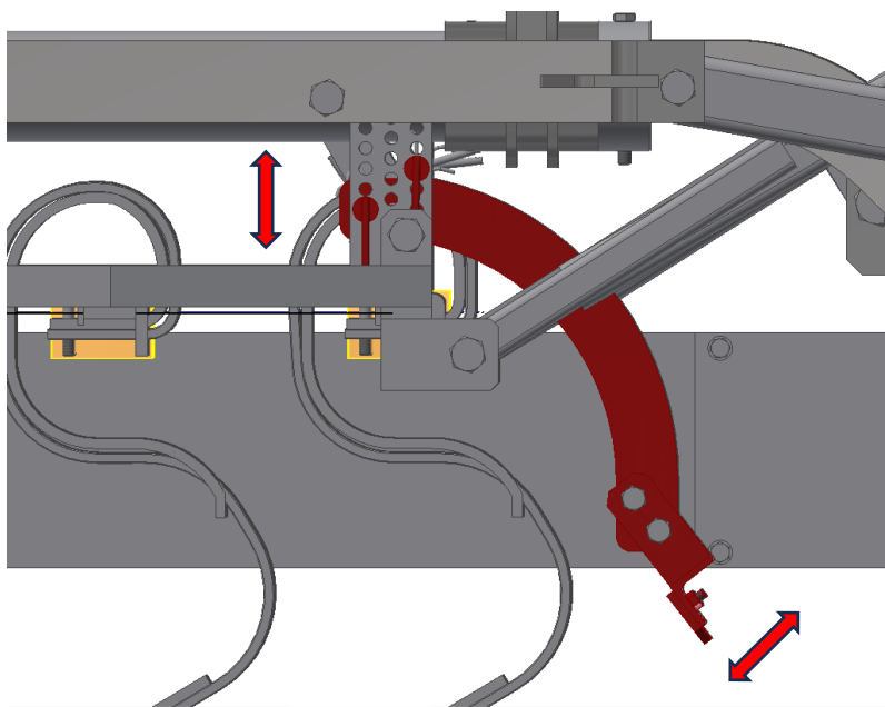
Rysunek 12 Regulacja włók wyrównującej
