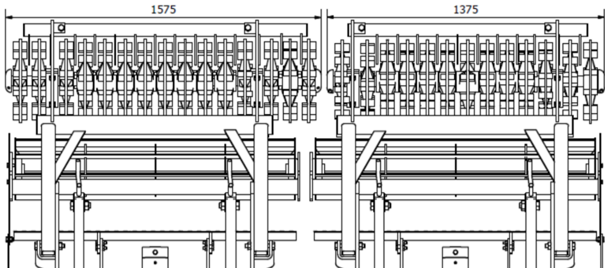
Rysunek 5 Ułożenie wałów kołeczkowych w FLEX 3.0
