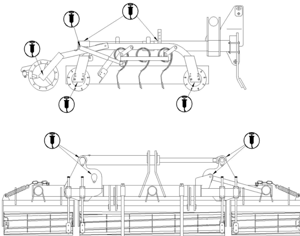
Rysunek 21 Punkty smarowania kultywatora przedsiewnego FLEX
