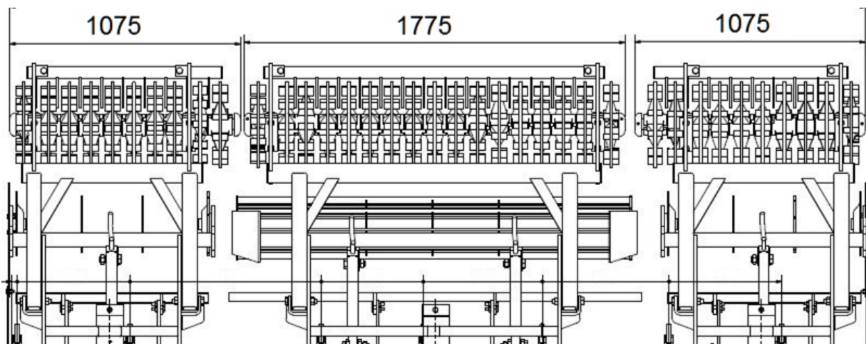
Rysunek 6 Ułożenie wałów kołeczkowych w FLEX 4.0H
