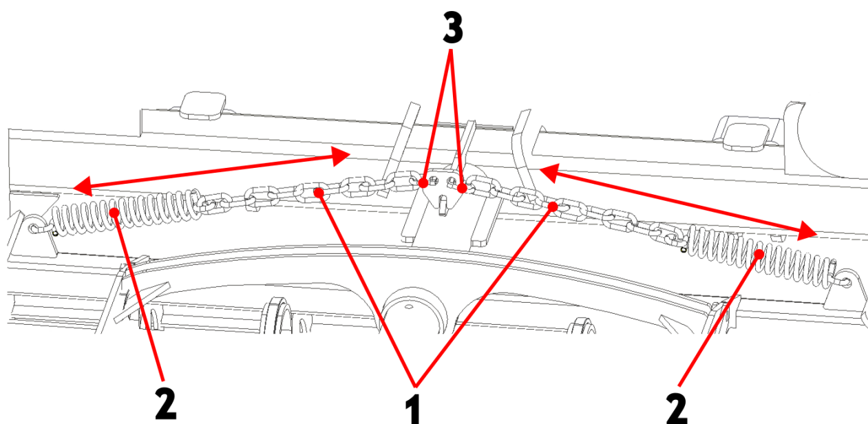
Rysunek 16 Odciagi łańcuchowo-sprężynowe (1 - łańcuch, 2 - sprężyna, 3 - szkło)
