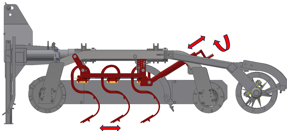
Rysunek 11 Regulacja głębokości pracy zębów kultywatora przedsiewnego FLEX.
