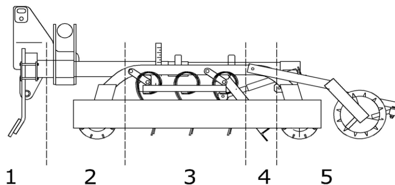
Rysunek 1 Sekcje robocze kultywatora przedsiewnego FLEX (1- spulchniacze śladów, 2- wał Ø350 mm krusząco wyrównujący, 3- sekcja zębów, 4- wółka wyrównująca, 5- sekcja wałów dogniatająco-kruszących Ø350 mm i kołeczkowy Ø400 mm)
