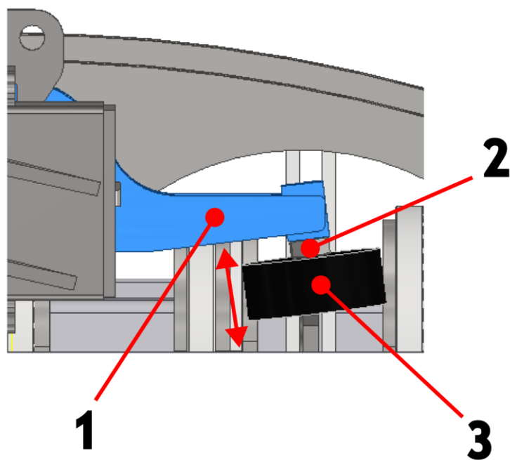
Rysunek 17 Budowa odboju (na przykładzie odboju pola bocznego) (1 - odbój, 2 - nakrętka kontrująca, 3 - odbój gumowy)
