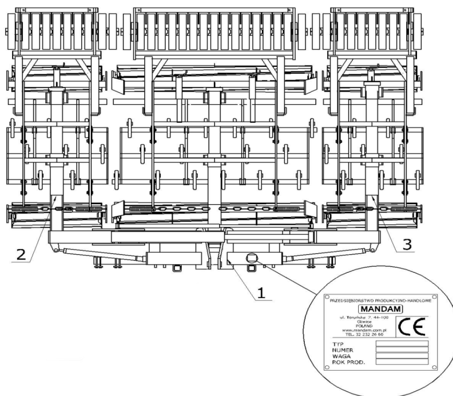
Rysunek 2 Widok kultywatora przedsiewnego FLEX H z miejscem mocowania tabliczki znamionowej (1- rama środkowa, 2- rama prawa z sekcjami roboczymi, 3- rama lewa z sekcjami roboczymi)
