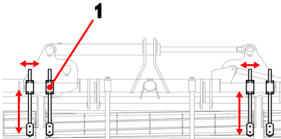
Rysunek 13 Regulacja głębokości pracy i rozstawu spulchniaczy śladów (1 - spulchniacz śladów)
