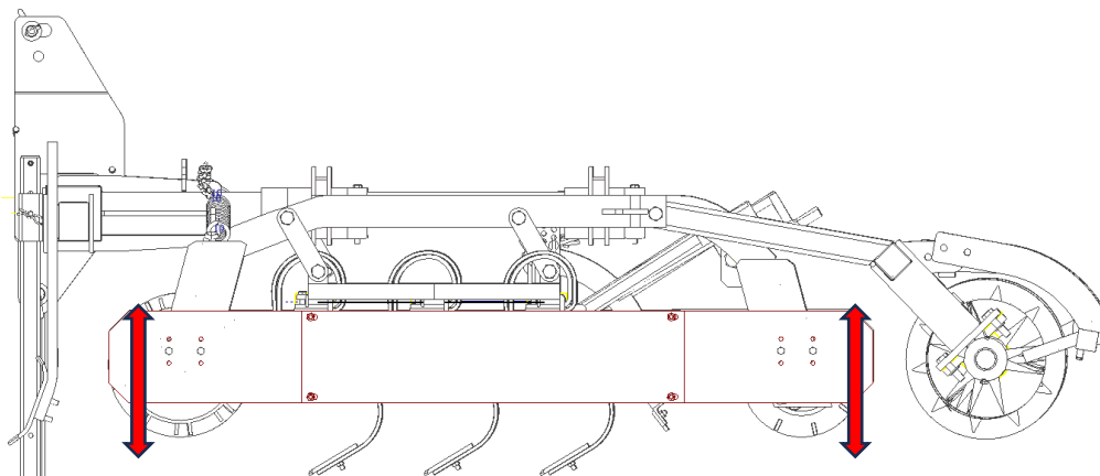
Rysunek 14 Regulacja ustawienia wysokości ekranów bocznych
