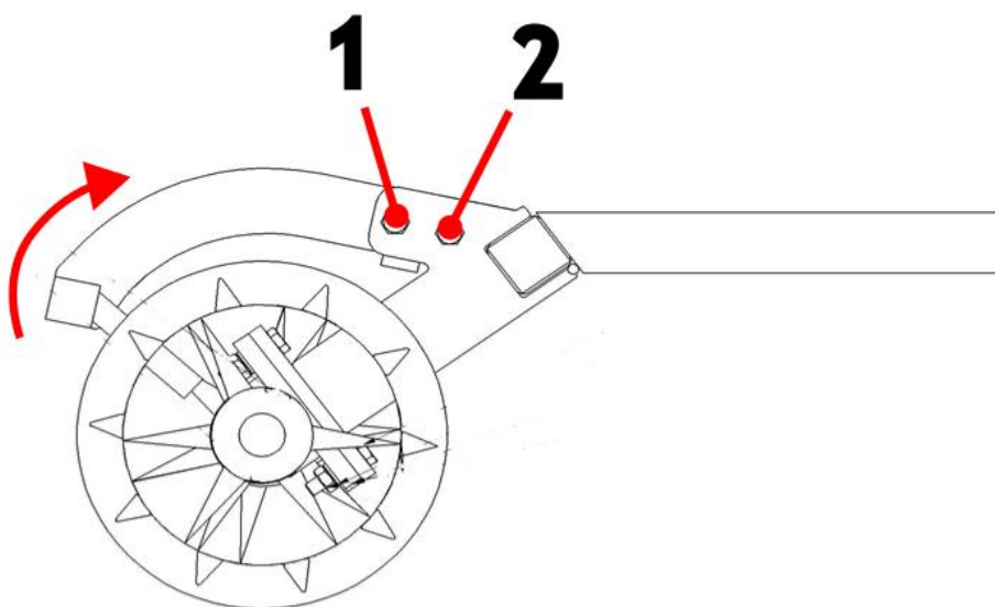
Rysunek 15 Odchylenie grzebienia oczyszczającego wału kołeczkowego (1 i 2 - śruby mocowania grzebienia oczyszczającego)
