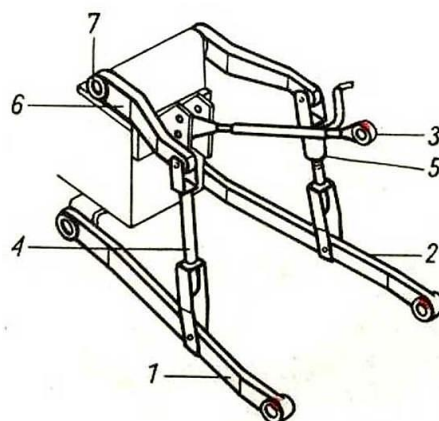
Rysunek 9 Trzypunktowy układ zawieszenia TUZ ciągnika: 1,2 - ciągnia dolne, 3 - łącznik górny, 4 - wieszak lewy, 5 - wieszak prawy o regulowanej długości, 6 - ramię podnośnika, 7 - wał podnośnika
