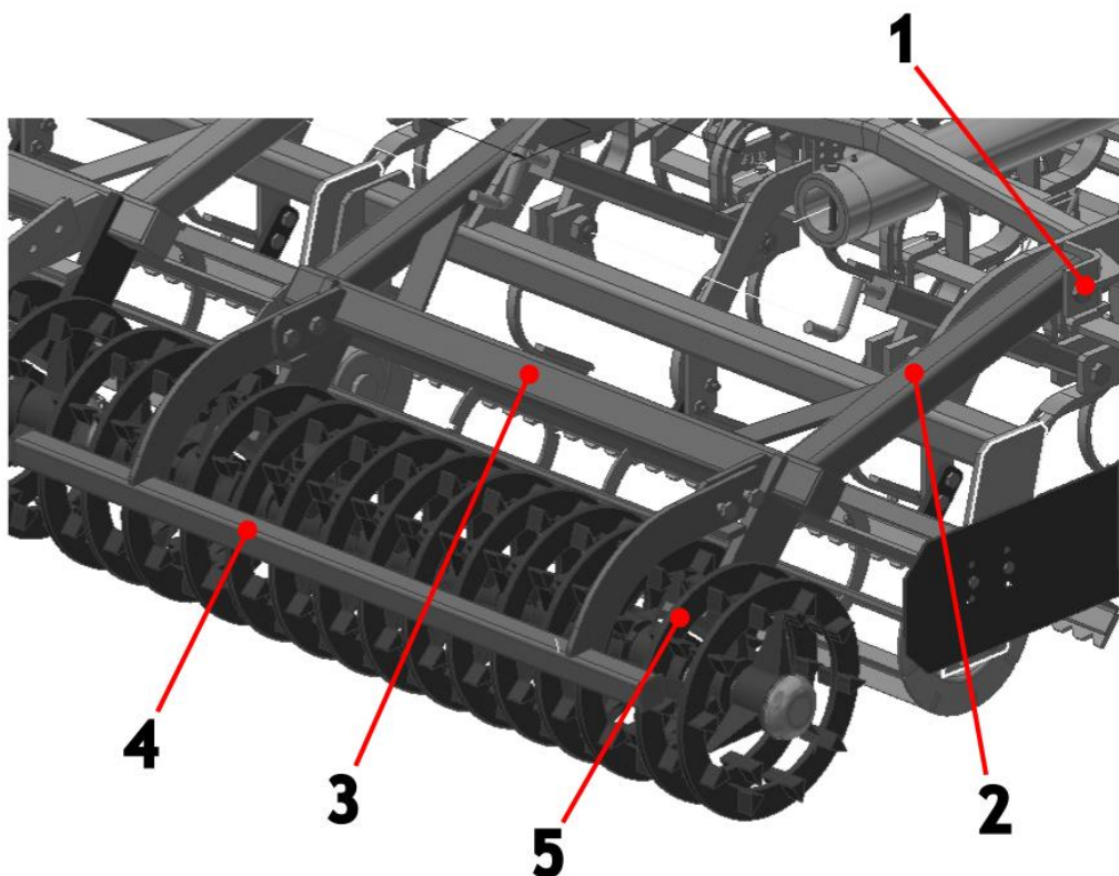
Rysunek 4 Widok montażu wału kołeczkowego do kultywatora FLEX (1 - śruby montażowe ramion do ramy kultywatora, 2 - ramiona obejmą wału, 3 - obejmą wału, 4 - złącznik wału, 5 - wał kołeczkowy)
