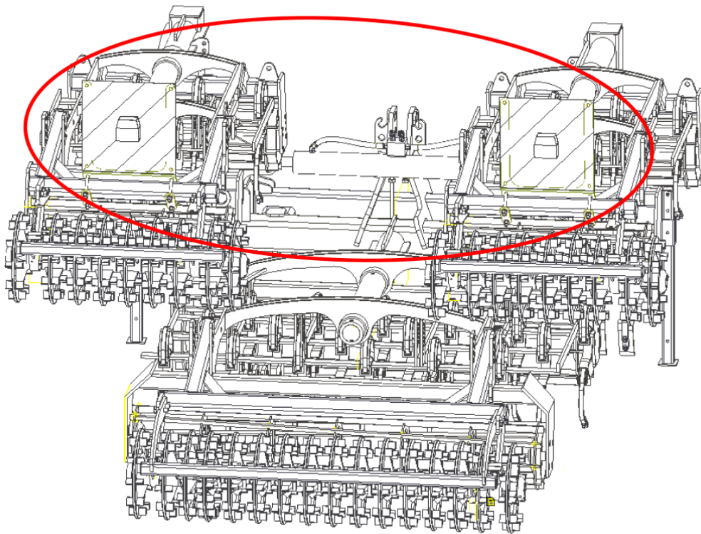
Rysunek 19 Zespół oświetlenia tylnego wraz z jego usytuowaniem dla kultywatora przedsiewnego FLEX 4,0 H
