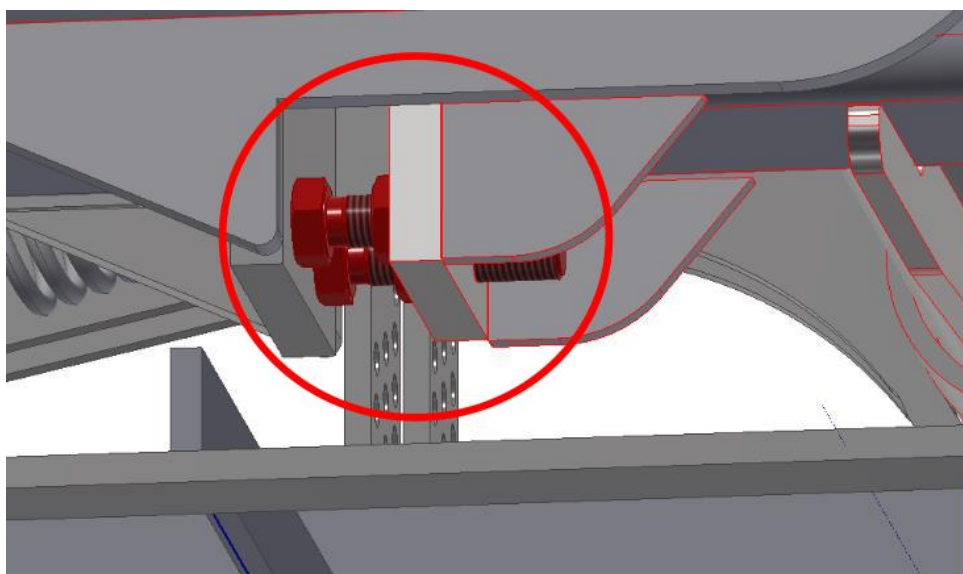
Rysunek 18 Śruby do regulacji poziomowania skrzydeł kultywatora
