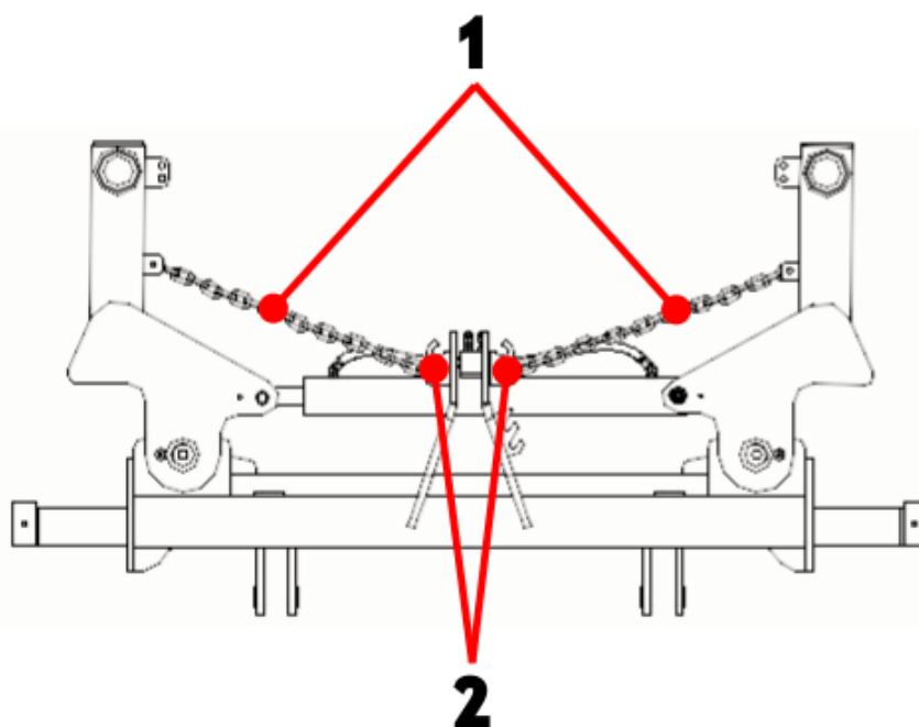
Rysunek 10 Łańcuchowe zabezpieczenie przed rozłożeniem kultywatora podczas transportu (1 - łańcuchy zabezpieczające, 2 - szkle)
