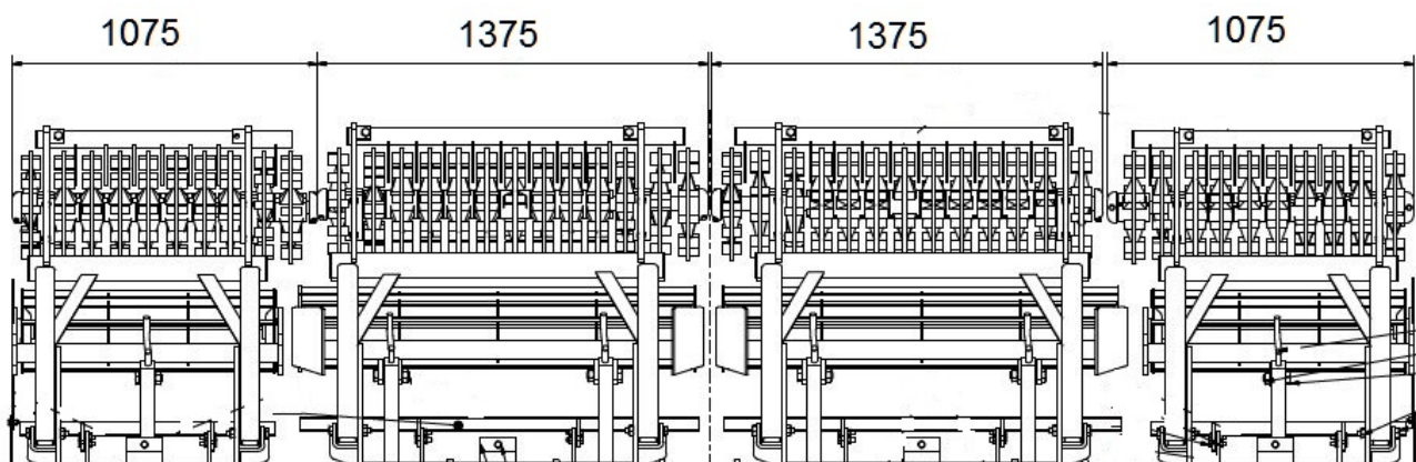
Rysunek 7 Ułożenie wałów kołeczkowych w FLEX 5.0H
