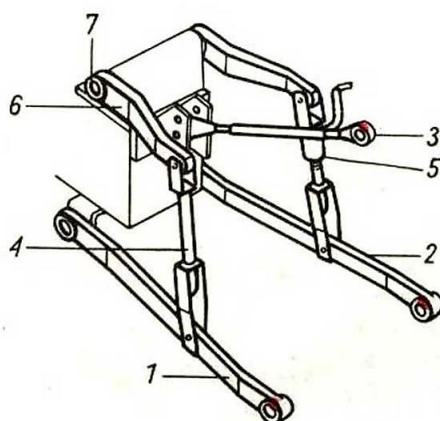
Rys. 18 Trzypunktowy układ zawieszenia TUZ ciągnika: 1, 2 - cięgła dolne, 3 - łącznik górny, 4 - wieszak lewy, 5 - wieszak prawy o regulowanej długości, 6 - ramię podnośnika, 7 - wał podnośnika.
