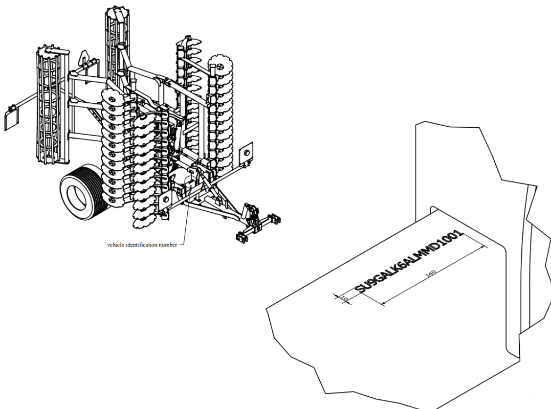
Rys. 2 Lokalizacja umieszczenia numeru identyfikacyjnego VIN na maszynie.
