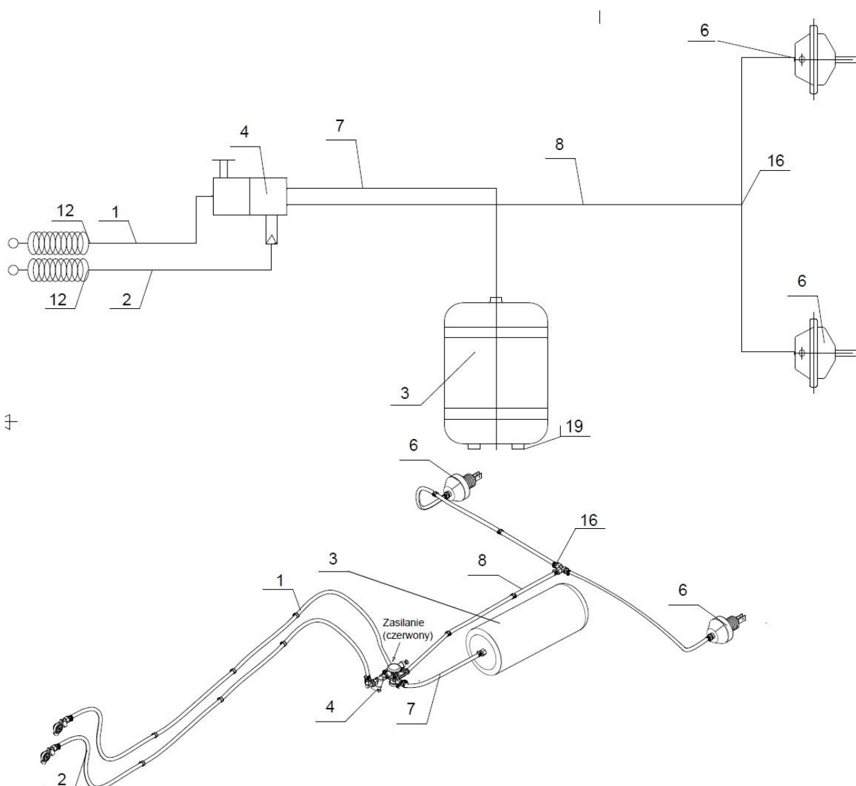
Rys.3 Schemat pneumatyczny brony BTH z dyszlem BTH-D: 1 - złącze z przewodem spiralnym (czerwone), 2 - złącze z przewodem spiralnym (żółte), 3 - zbiornik powietrza 40L, 4 - zawór sterujący przyciepą, 6 - siłownik membranowy 24", 7-8 - przewód gumowy powietrzny, 12- redukcja, 16 - trójnik M22, 19 - korek zbiornika.
