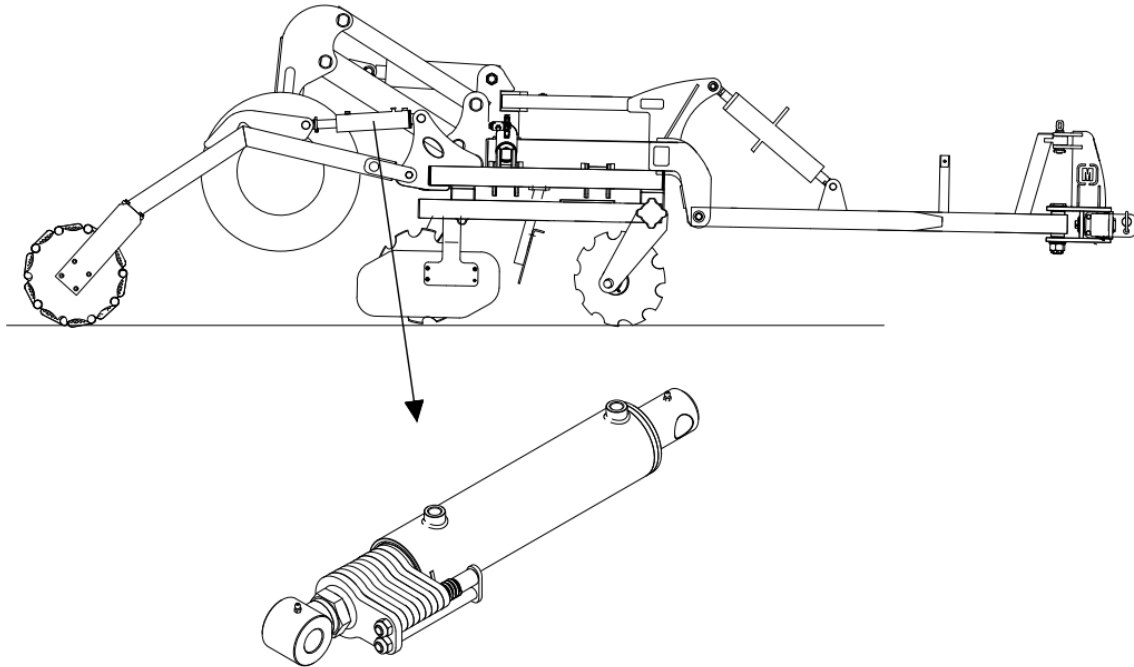
Rys. 25 Siłownik z zapadkami założonymi na tłoczysku w celu regulacji głębokości roboczej.
