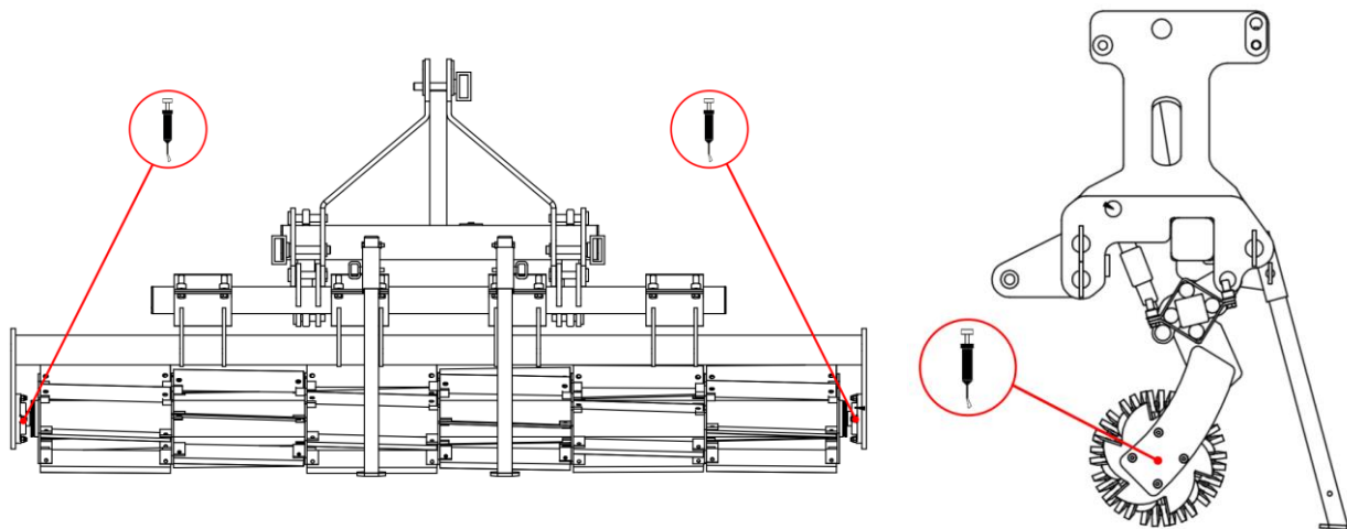
Rysunek 8 Punkty smarowania wału nożowego (wersja nie składana hydraulicznie)
