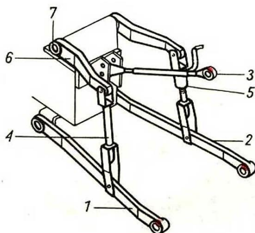
Rysunek 6 Trzypunktowy układ zawieszenia TUZ ciągnika: 1,2 - cięgła dolne, 3 - łącznik górny, 4 - wieszak lewy, 5 - wieszak prawy o regulowanej długości, 6 - ramię podnośnika, 7 - wał podnośnika
