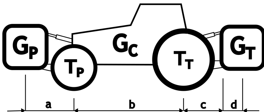
Rysunek 5 Schemat oznaczeń obciążeń ciągnika
