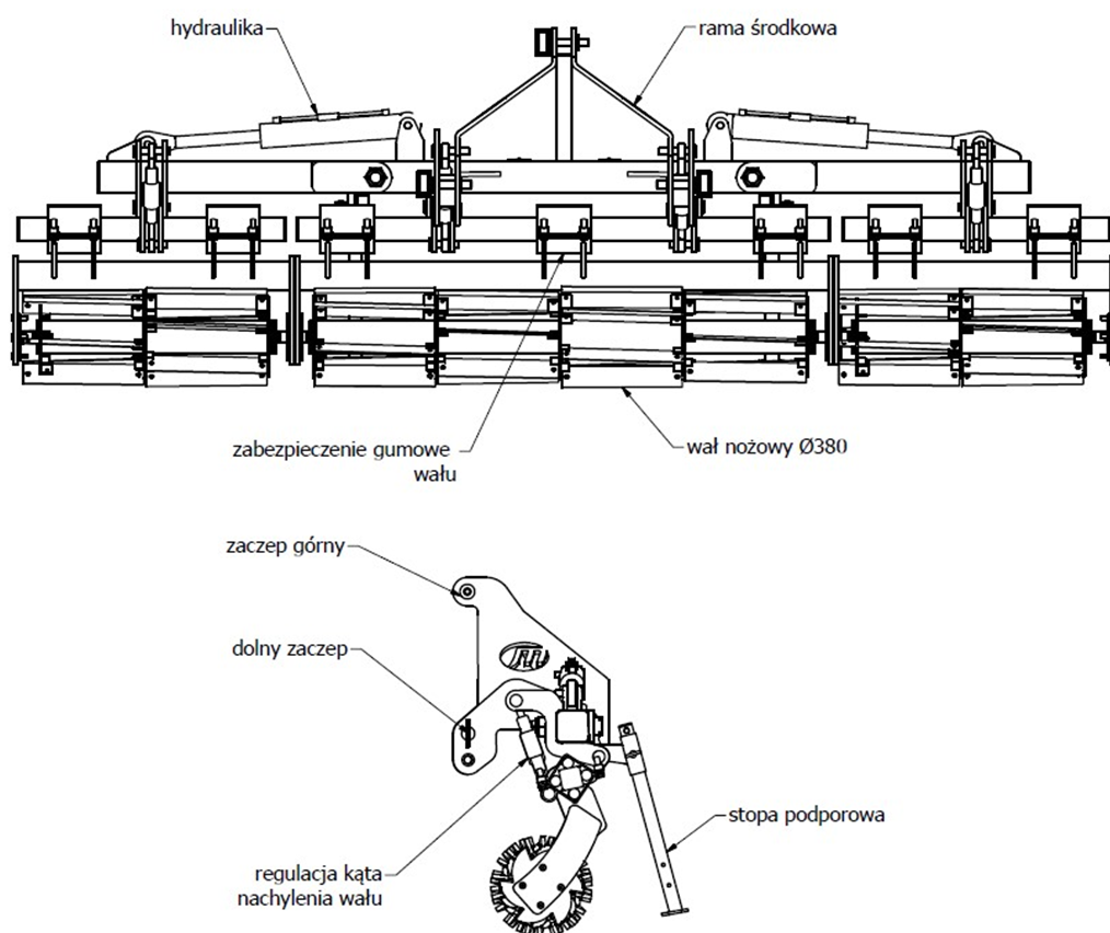
Rysunek 3 Budowa wału nożowego składanego hydraulicznie na przykładzie wersji o szerokości 4,0m
