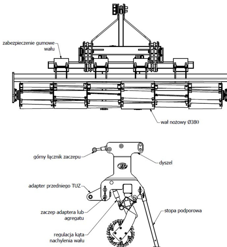
Rysunek 2 Budowa wału nożowego na przykładzie wersji o szerokości 3m.
