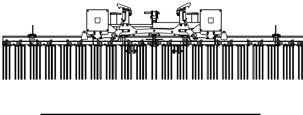
Rys. 13 Widok na maszynę w momencie zakończenia sekwencji otwierania skrzydeł. Ramiona maszyny są całkowicie otwarte.
