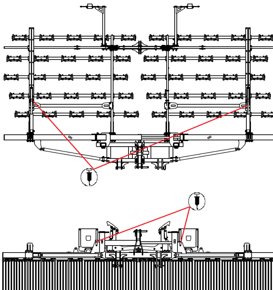
Rys. 15. Punkty smarowania Łamacza słomy MBS.
