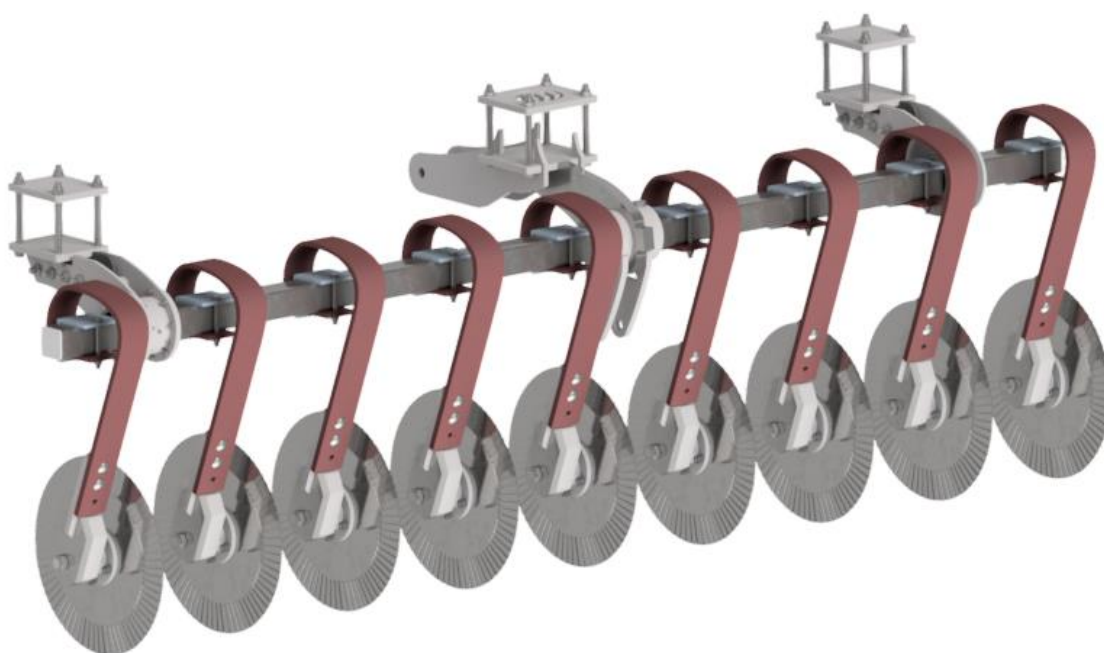
Rys. 6 Zespół belki talerzy.
