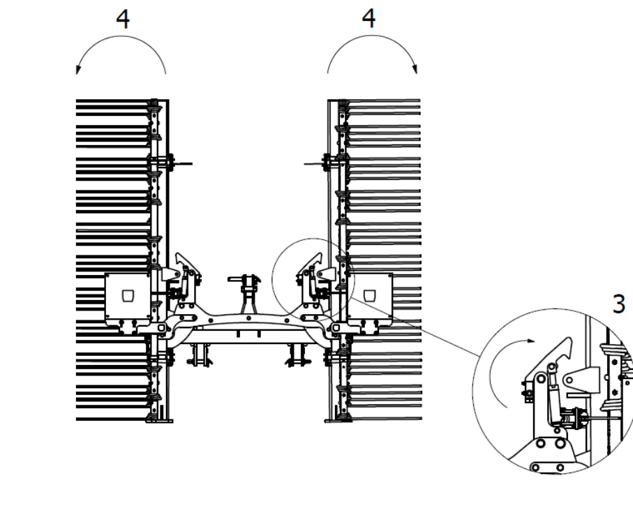
Rys. 11 Sekwencja otwierania maszyny: 3- uwolnienie haka mechanizmu hydraulicznej blokady skrzydeł 4- otwieranie skrzydeł maszyny.
