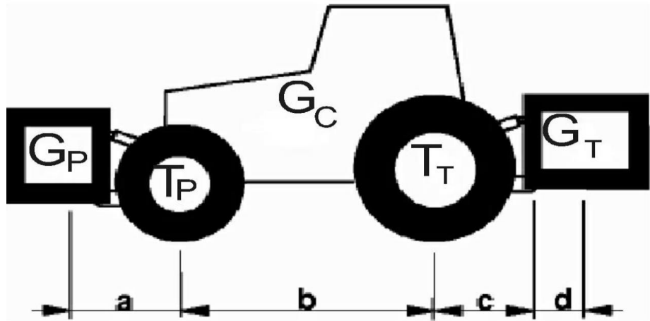
Fig. 2 Diagramme des désignations de charge du tracteur.
