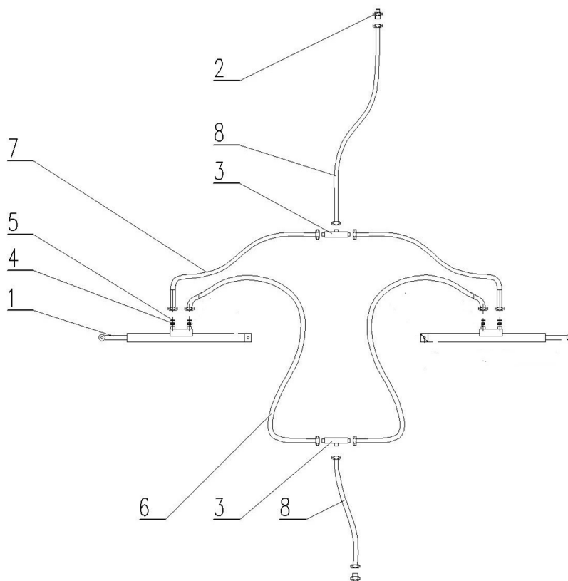
Fig. 14 Schéma du système hydraulique du SPEC HD : 1- vérin, 2- raccord rapide, 3- té, 4- bride, 5- rondelle en cuivre, 6- tuyau hydraulique 1 m, 7- tuyau hydraulique 0,7 m, 8- tuyau hydraulique 2,2 m.
