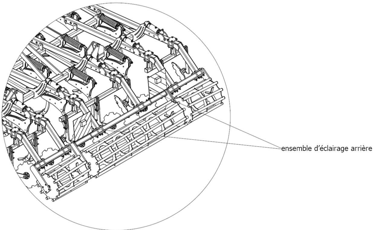
Fig. 13 Ensemble d'éclairage arrière et son emplacement.
