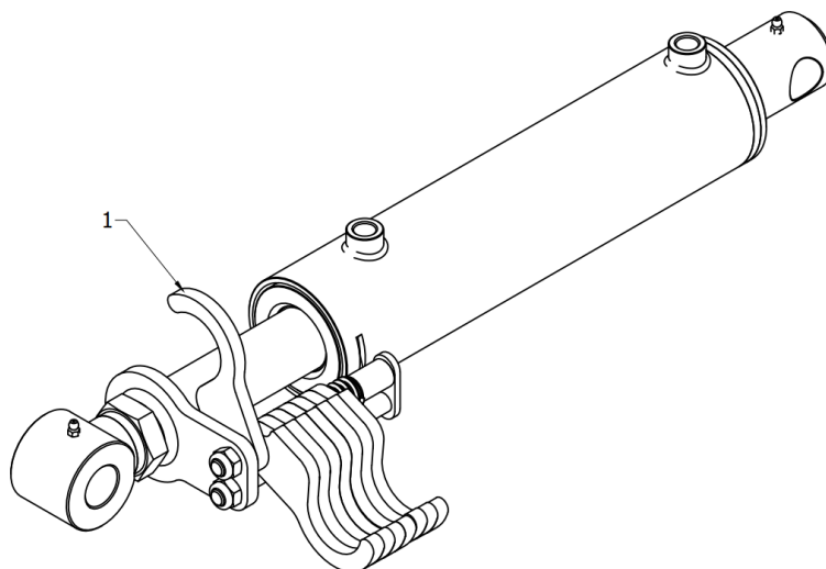
Fig. 11 Accrochage correct du premier (1) cliquet sur la tige de piston du vérin pour le réglage de la profondeur de travail de la machine.
