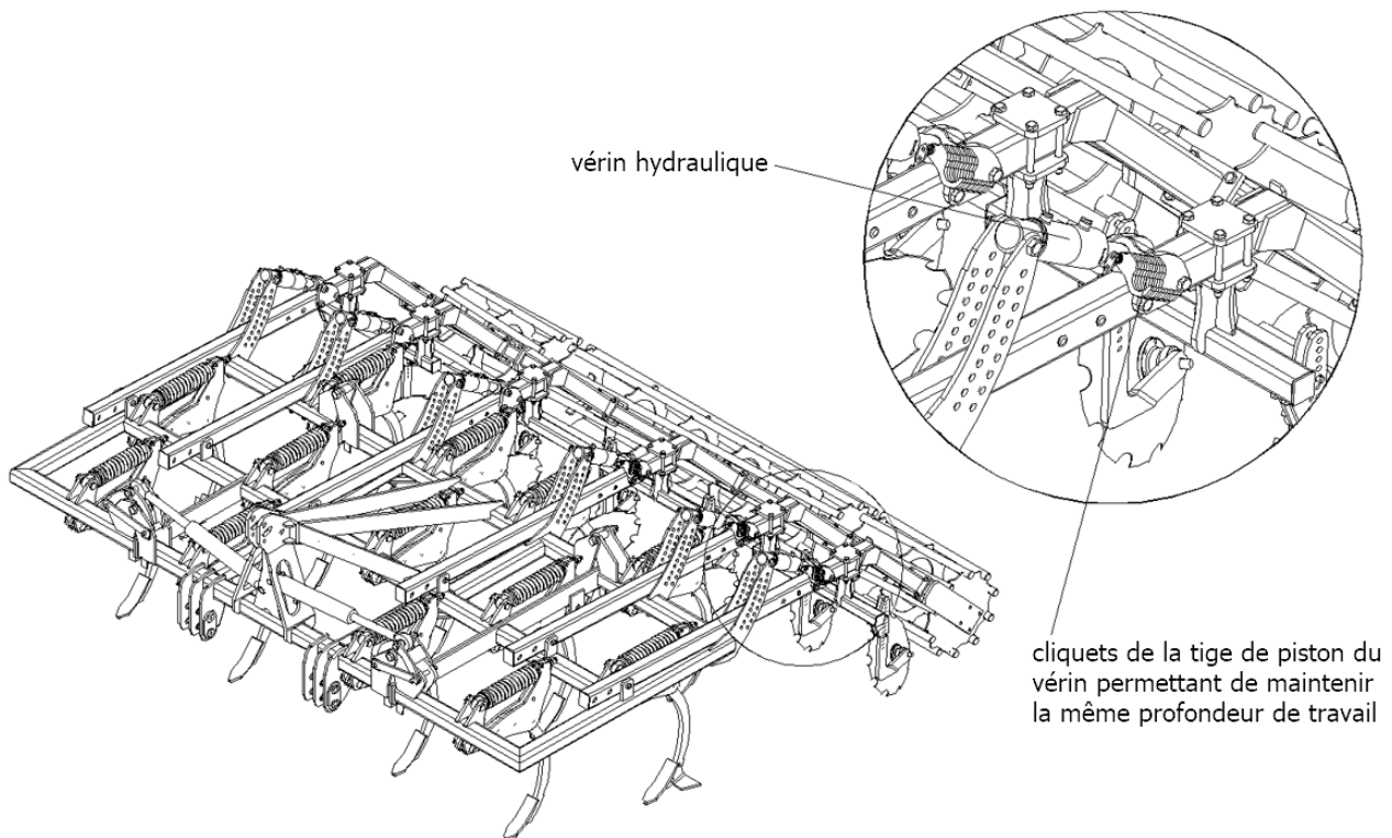
Fig. 10 Réglage hydraulique de la profondeur du rouleau.
