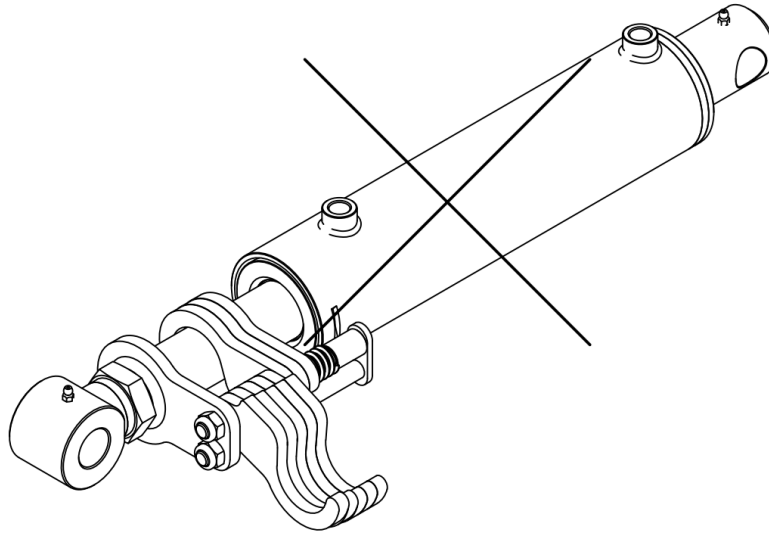
Fig. 12 Accrochage incorrect des cliquets sur la tige de piston du vérin. L'omission de cliquets entraîne une répartition inégale des forces agissant sur la tige de piston et peut conduire à un flambage de celle-ci et, en conséquence, à l'endommagement de l'ensemble du vérin. Ce mode de réglage est inadmissible!
