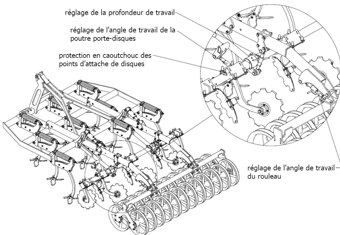
Fig. 9 Réglage mécanique de la profondeur du rouleau à l'aide des tendeurs.
