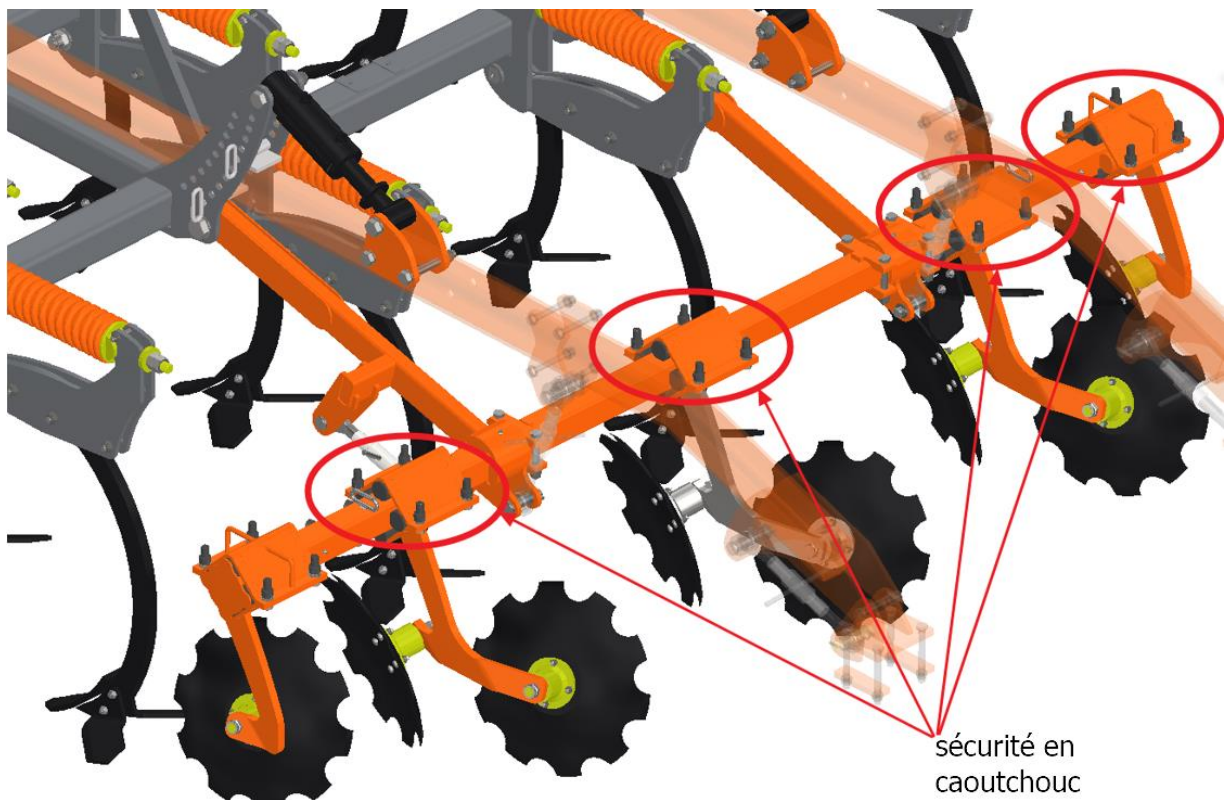
Fig.5 Poutre porte-disques à sécurité caoutchouc.
