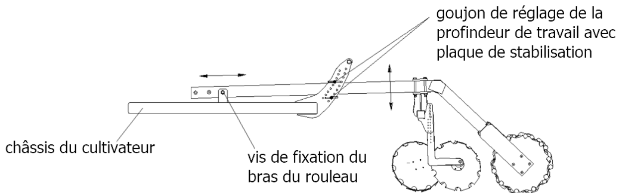
Fig. 8 Réglage de la profondeur et de l'écartement du rouleau.
