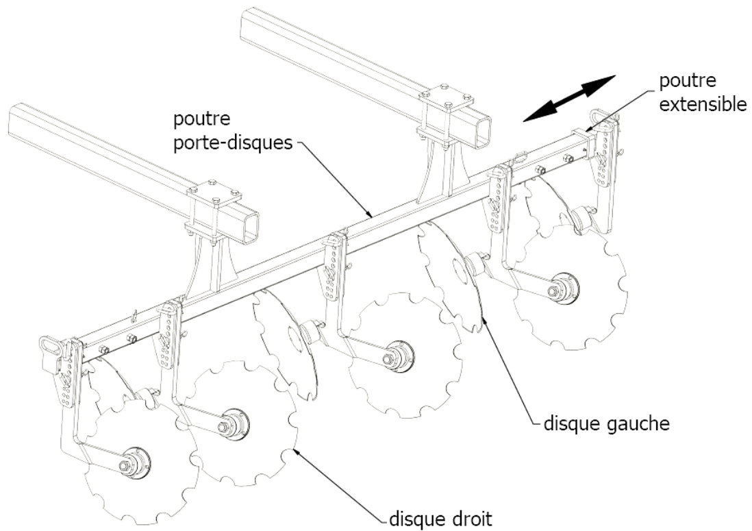
Fig. 4 Disposition des disques sur la poutre.
