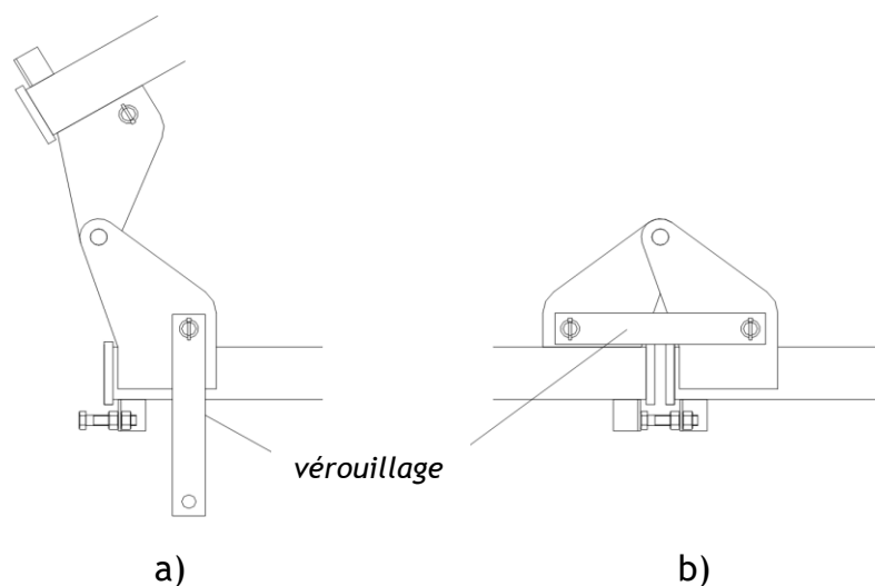
Fig. 7 Verrouillage en position de transport (fig. a), verrouillage en position de travail (fig. b).
