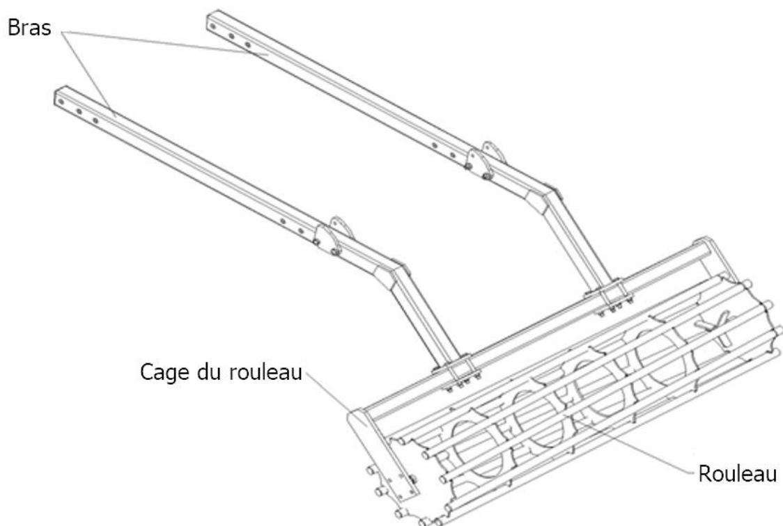
Fig. 3 Fixation des bras à la cage du rouleau-barre.
