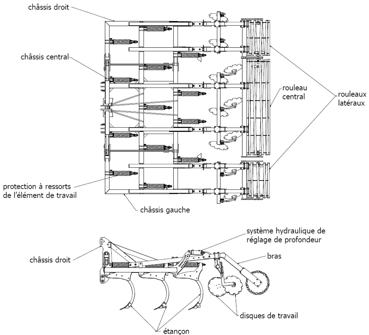
Fig.1 Cultivateur à dents SPEC HD 4.0 H.
