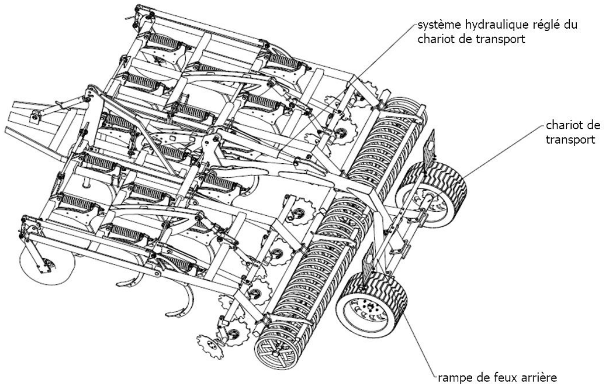
Fig. 15 Cultivateur SPEC HD équipé d'un chariot de transport (en option).
