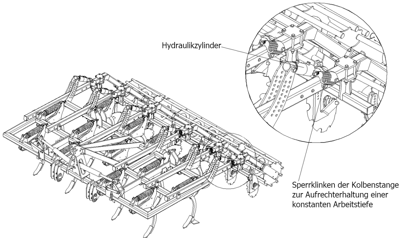
Abb. 10 Hydraulische Einstellung der Arbeitstiefe der Rohrwalze.
