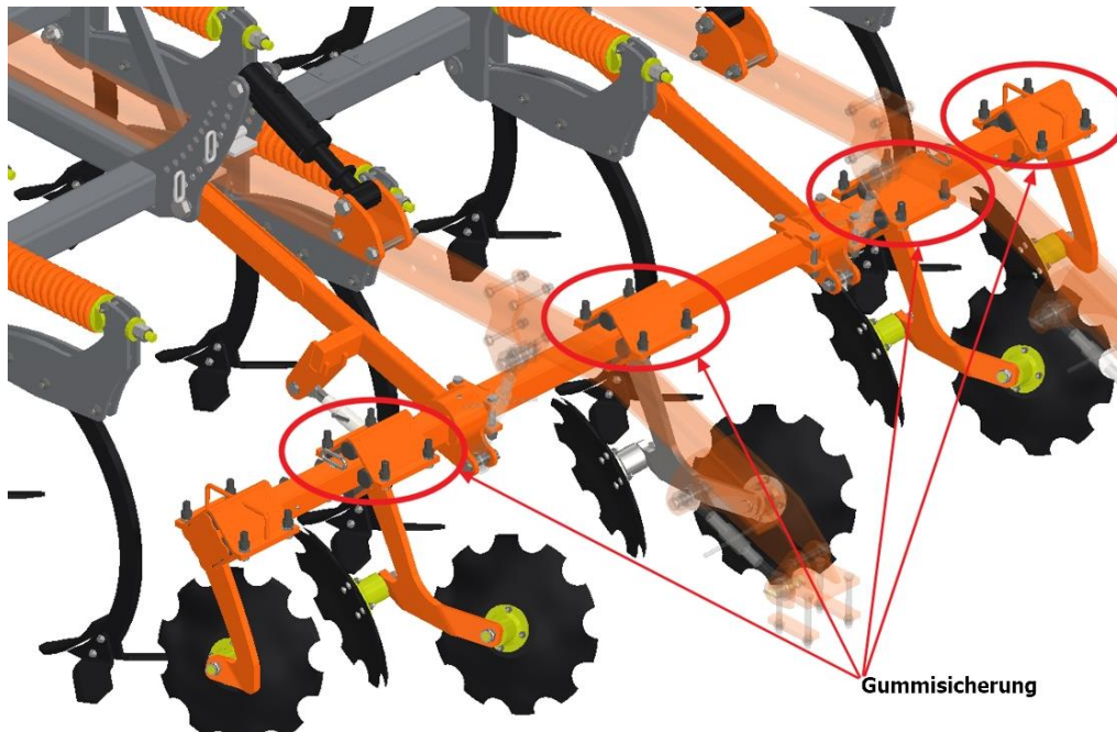
Abb.5 Tellerbalken mit Gummischutz.
