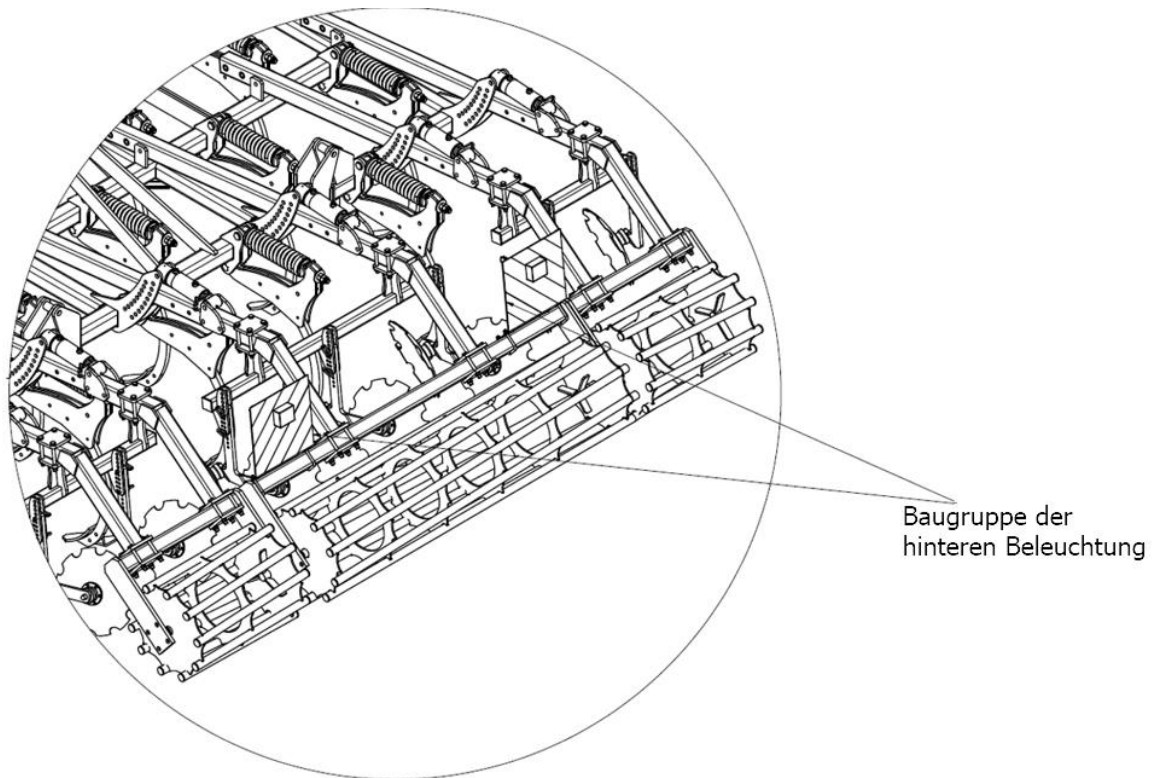
Abb. 13 Baugruppe der hinteren Beleuchtung und deren Anordnung.
