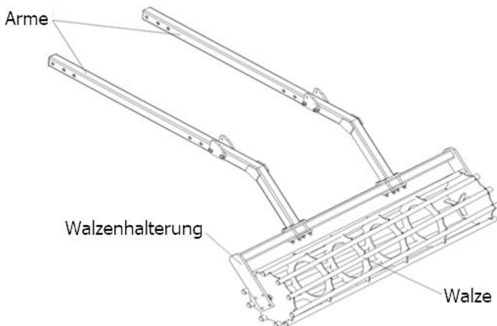
Abb. 3 Verbindung der Arme mit der Halterung der Walze.
