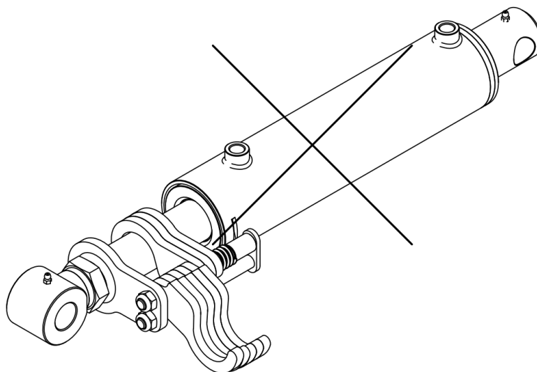
Abb. 12 Inkorrekte Anlegung der Sperrklinken an der Kolbenstange des Zylinders. Ein teilweiser Verzicht auf die Befestigung der Sperrklinken am Stellantrieb führt zu einer ungleichmäßigen Verteilung der auf die Kolbenstange wirkenden Kräfte und kann zu einem Ausknicken der Kolbenstange und damit zu einer Beschädigung der gesamten Zylinderbaugruppe führen. Diese Art der Regulierung ist unzulässig!
