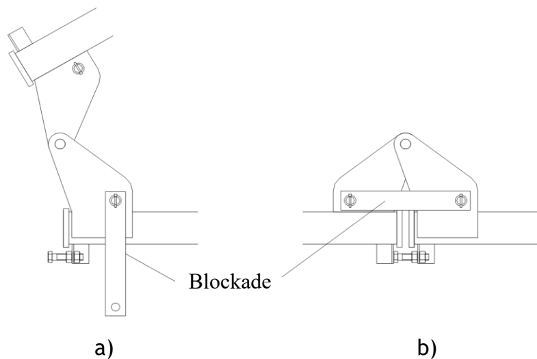
Abb. 7 Sperre in Transportstellung (Abb. a), Sperre in Arbeitsstellung (Abb. b).
