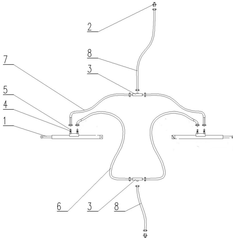
Abb. 14 Schema des Hydrauliksystems des Grubbers SPEC HD: 1- Zylinder, 2- Schnellkupplung, 3- T-Stück, 4- Drosselscheibe, 5- Kupferunterlegscheibe, 6- Hydraulikleitung 1m, 7- Hydraulikleitung 0,7m, 8- Hydraulikleitung 2,2m.
