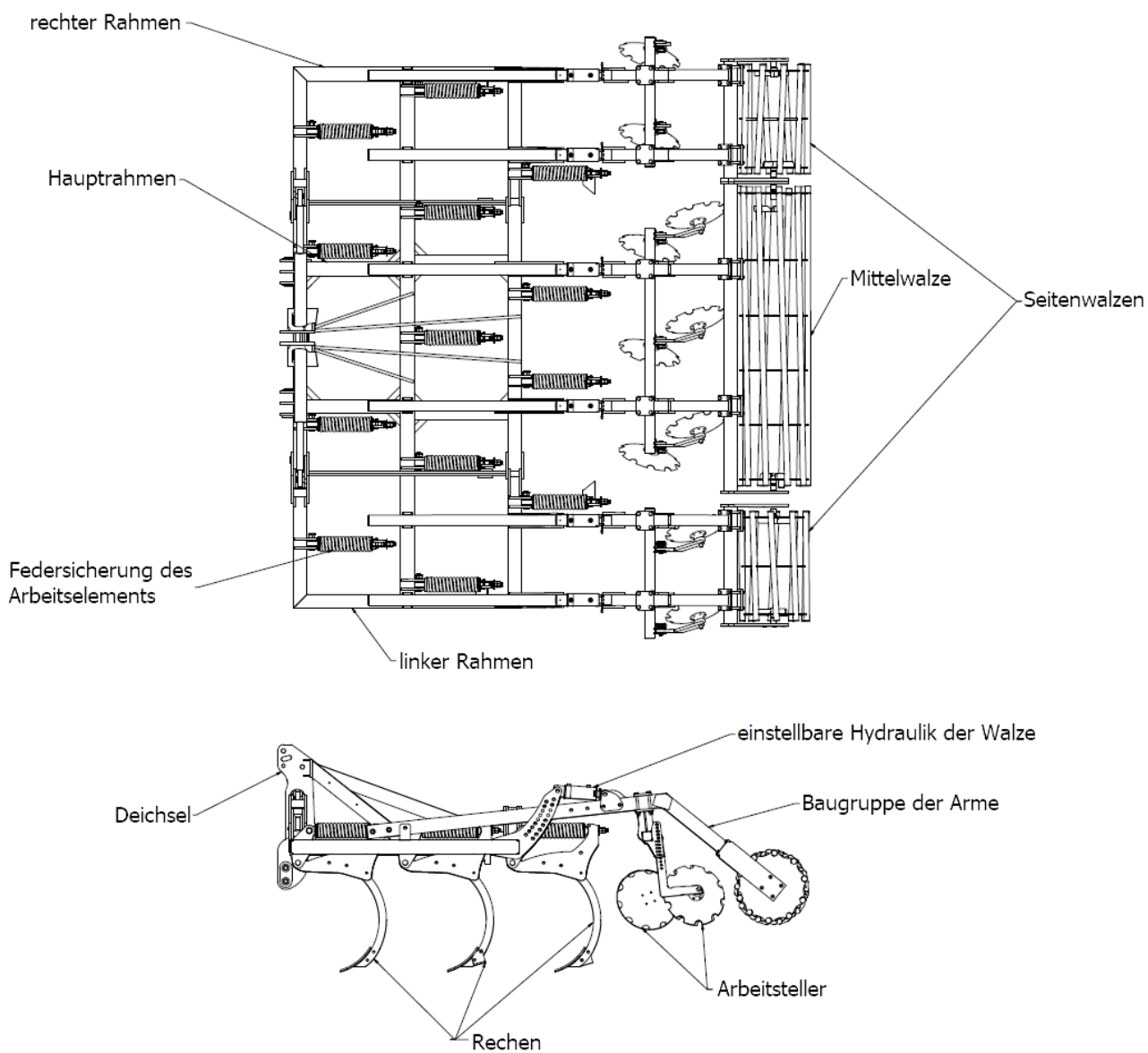
Abb.1 Mulchgrubber SPEC HD 4.0 H.
