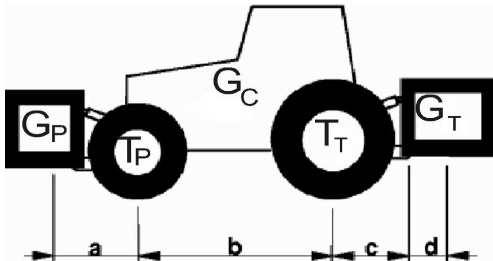
Abb. 2 Schema Lastkennzeichnungen des Traktors
