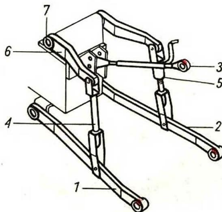
Abb. 6 Dreipunktaufhängung des Traktors: 1, 2 - Unterlenker, 3 - Oberlenker, 4 - linke Hubstange, 5 - Höhenverstellbare rechte Hubstange, 6 - Hubarm, 7 - Welle des Hebers
