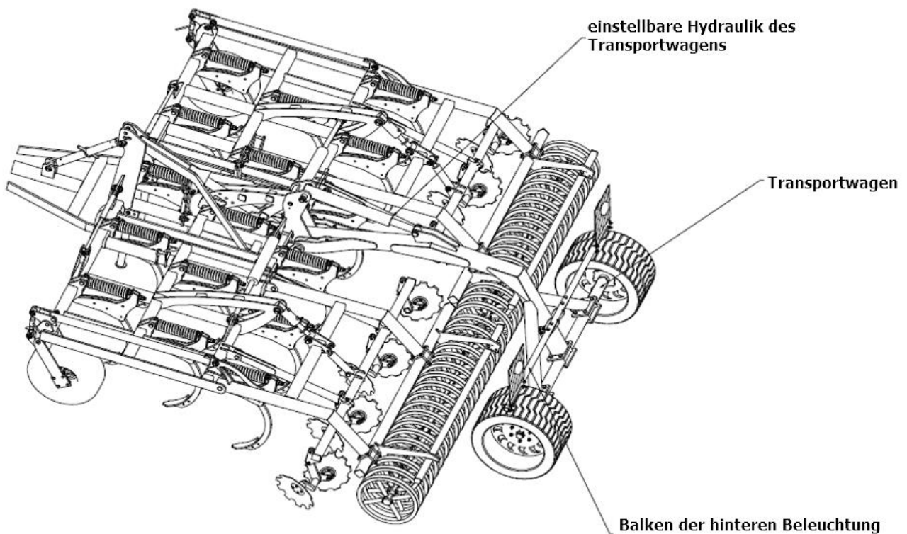
Abb. 15 Grubber SPEC HD mit einem Transportwagen (Option).
