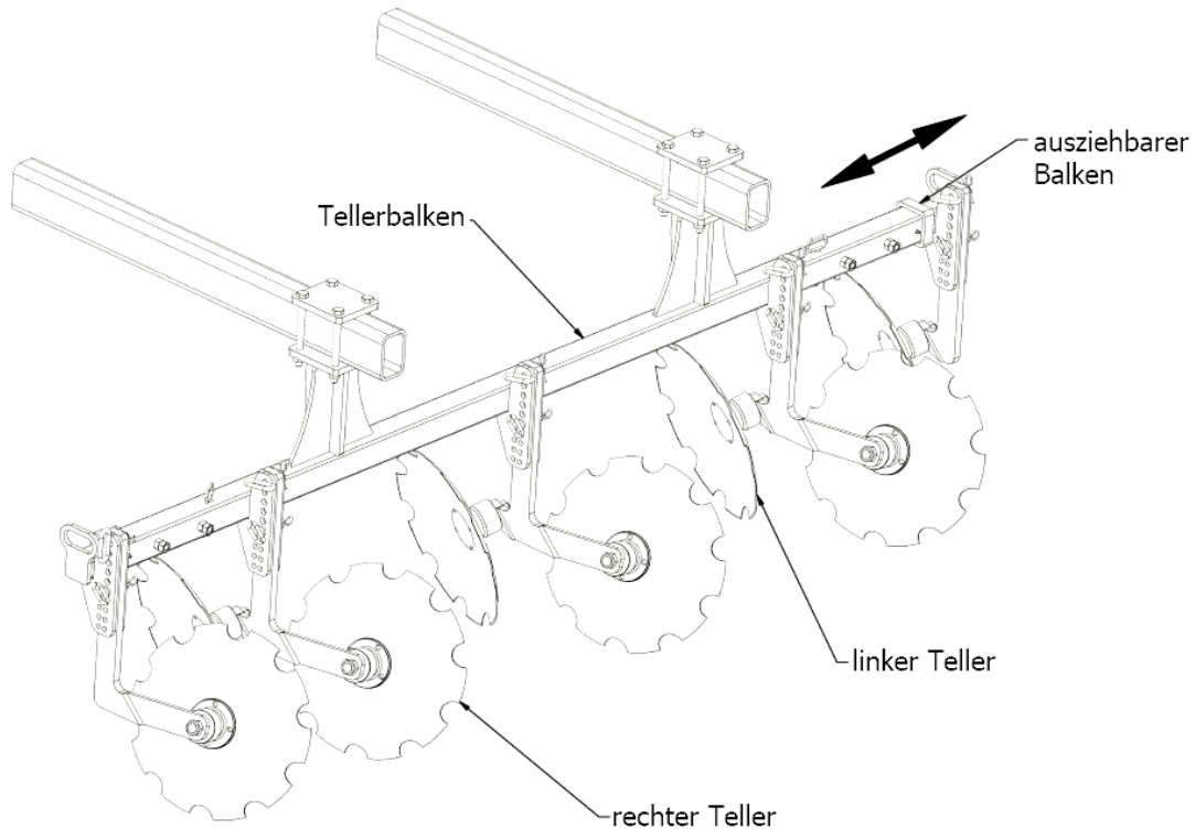
Abb. 4 Verteilung der Teller auf dem Balken.
