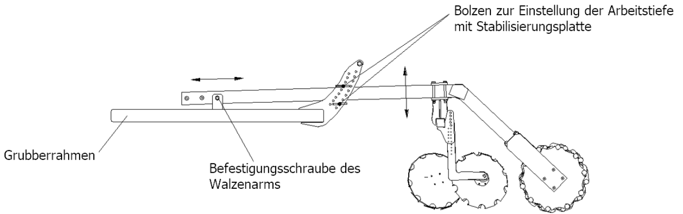
Abb. 8 Einstellung von Tiefe und Abstand der Rohrwalze.
