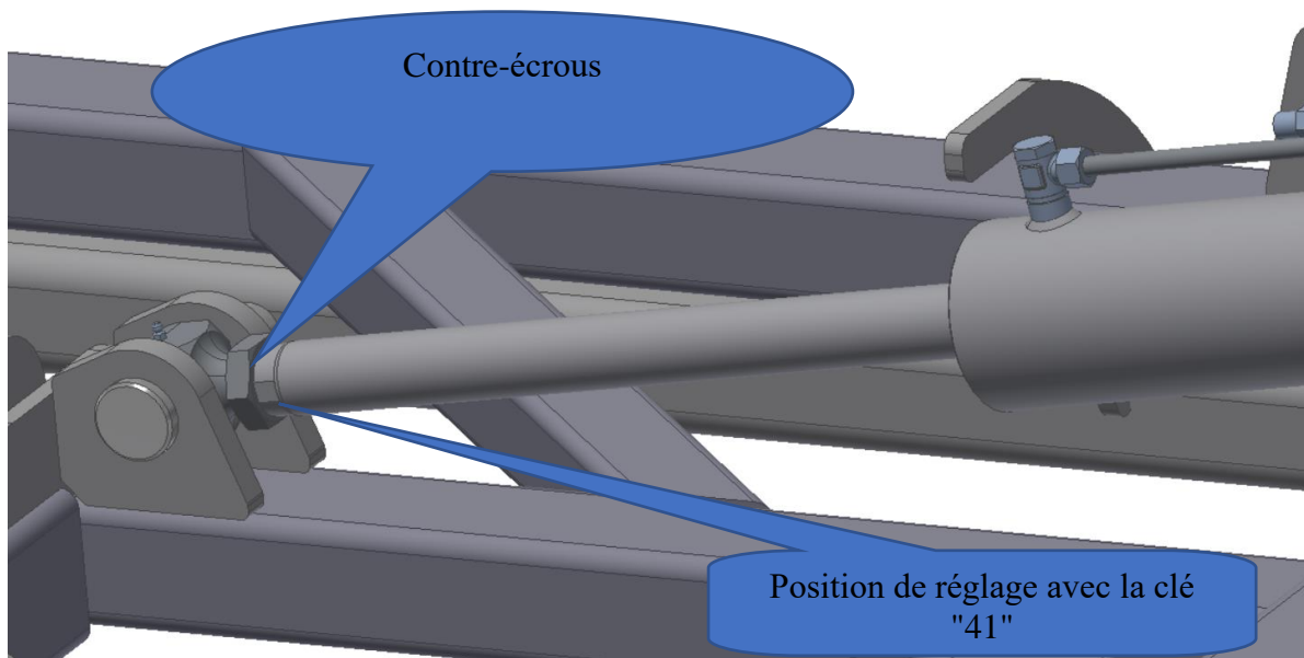
Fig. 17 Vue du vérin avec écrou pour la mise à niveau de la machine.
