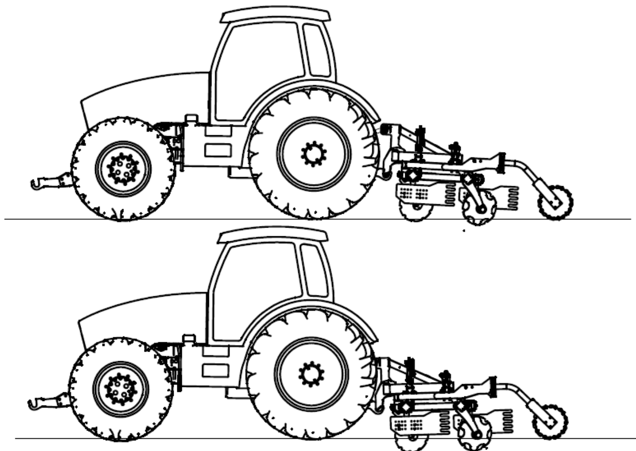
Fig. 13 Réglages incorrects de la machine.
