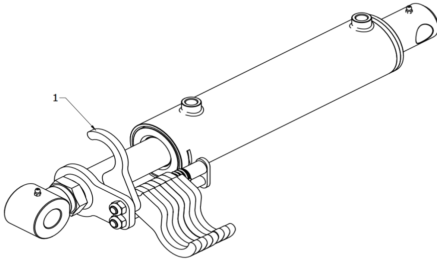
Fig. 19 Manière correcte de placer le premier (1) cliquet sur la tige de piston du cylindre pour régler la profondeur de travail de la machine.
