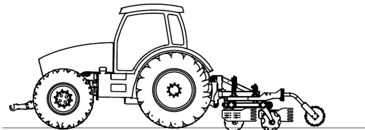
Fig. 12 Machine correctement positionnée et parallèle au sol.
