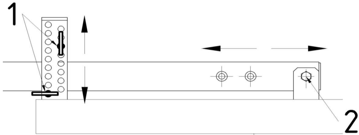
Fig. 18 Réglage de la profondeur et de l'écartement du rouleau : 1 - boulons de réglage de la profondeur de travail, y compris la plaque de stabilisation ; 2 - vis de fixation des bras du rouleau.
