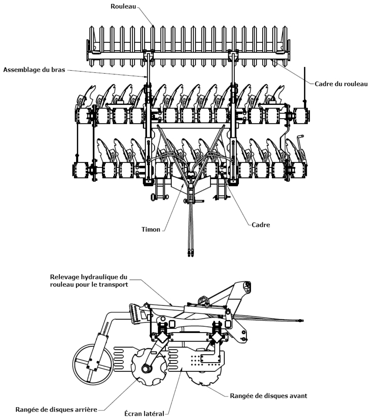
Fig.2 Le déchaumeur à disques GAL-E.
