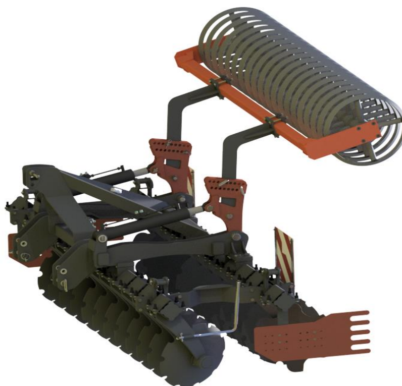
Fig. 3 Le déchaumeur à disques GAL-E avec rouleau relevé.
