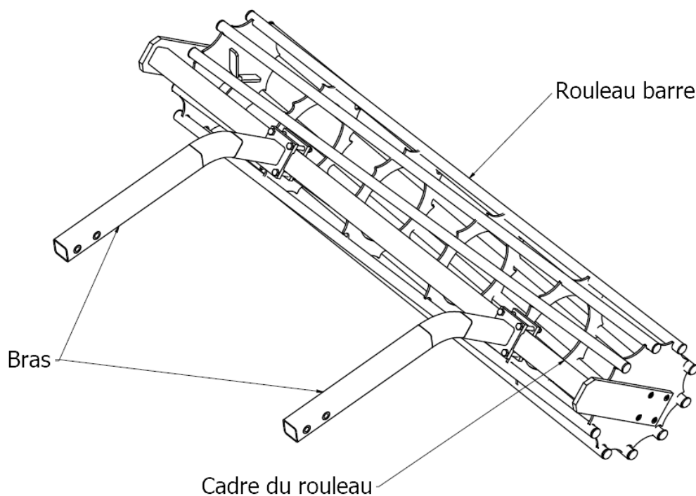
Fig. 5 Raccordement des bras à la fixation du rouleau.
