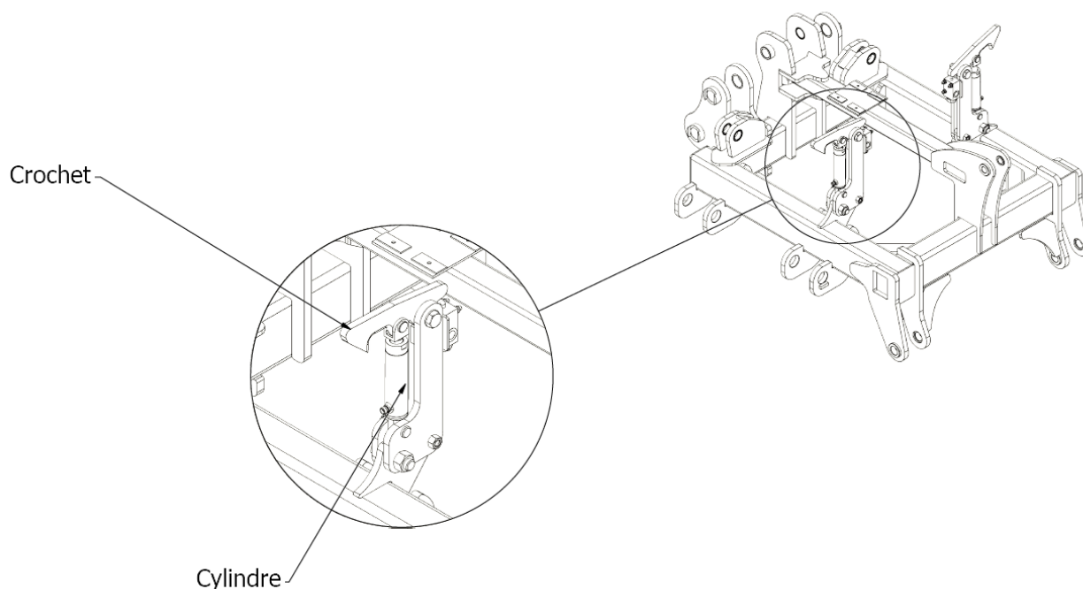
Fig. 7 Châssis central avec un verrouillage automatique des bras latéraux.
