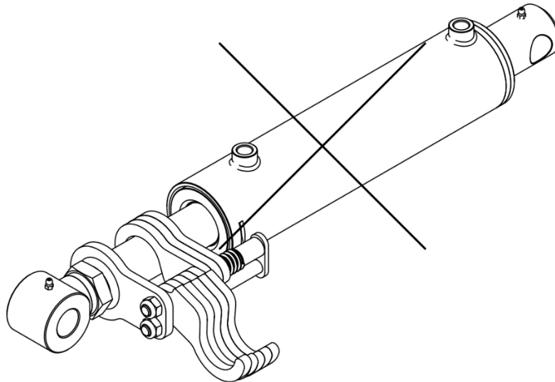
Fig. 20 Installation incorrecte des cliquets sur la tige du piston du vérin. L'omission partielle de la fixation des cliquets à l'actionneur entraîne une répartition inégale des forces agissant sur la tige du piston et peut conduire à un flambage de la tige du piston et endommager l'ensemble du vérin. Une telle installation des cliquets est inadmissible !
