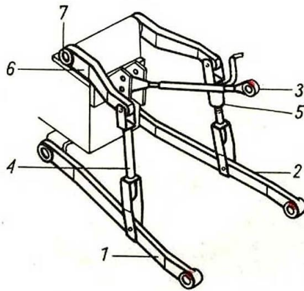
Fig. 2 Attelage trois-points du tracteur : 1, 2 - barres inférieures, 3 - tige de liaison supérieur, 4 - chandelle gauche, 5 - chandelle droite réglable, 6 - bras de relevage, 7 - arbre de relevage
