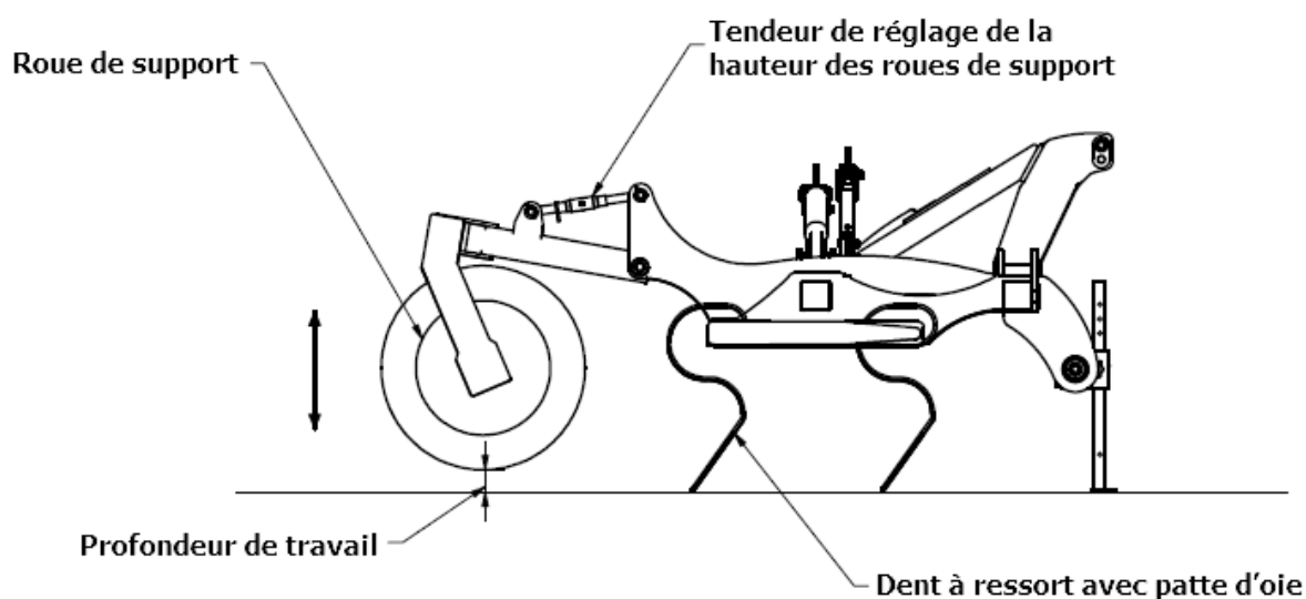
Fig. 8 Réglage de la profondeur de travail.
