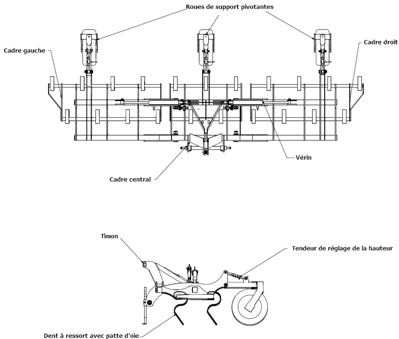
Fig. 1 Structure du cultivateur FRONT.
