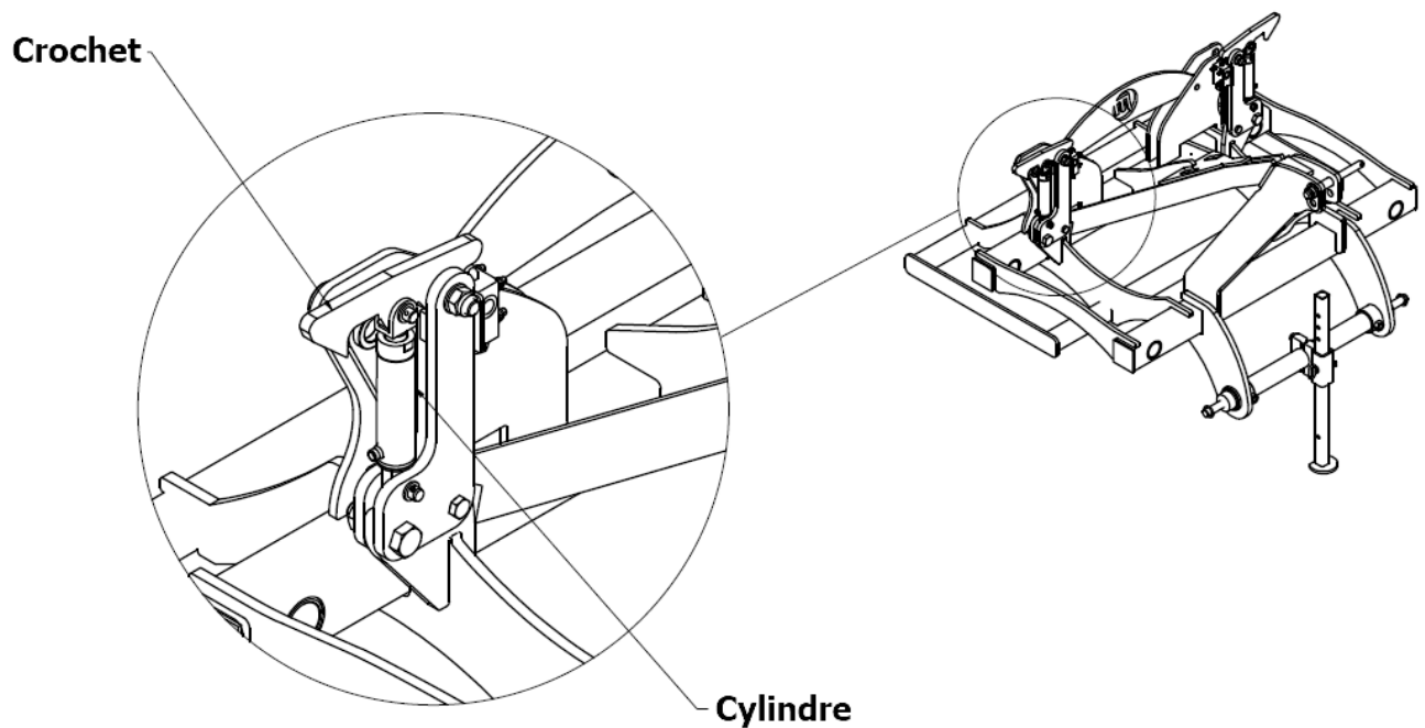
Fig. 3 Châssis central avec un verrouillage automatique des bras latéraux.
