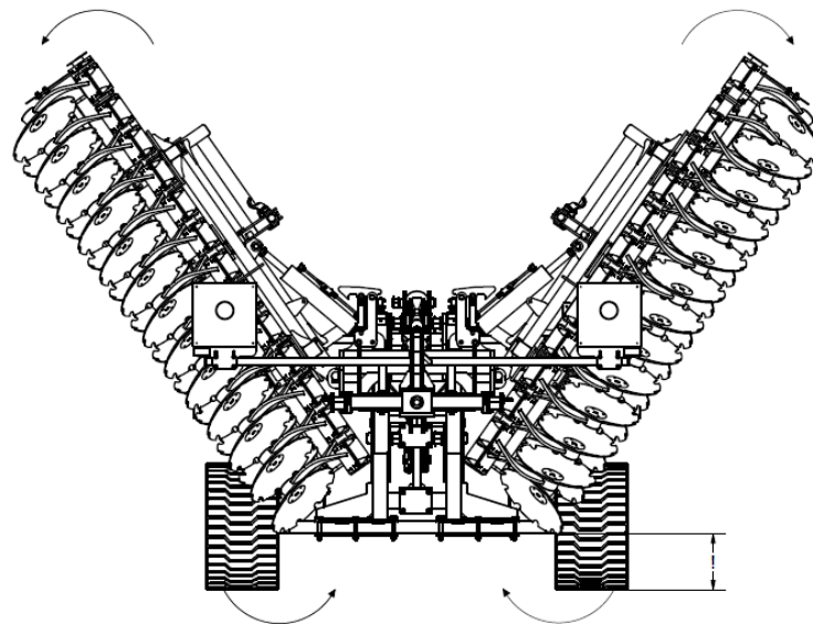
Rys. 7 Sekwencja otwierania maszyny: otwieranie maszyny ze zwróconą szczególną uwagę na wysokość końców ramion od podłoża.
