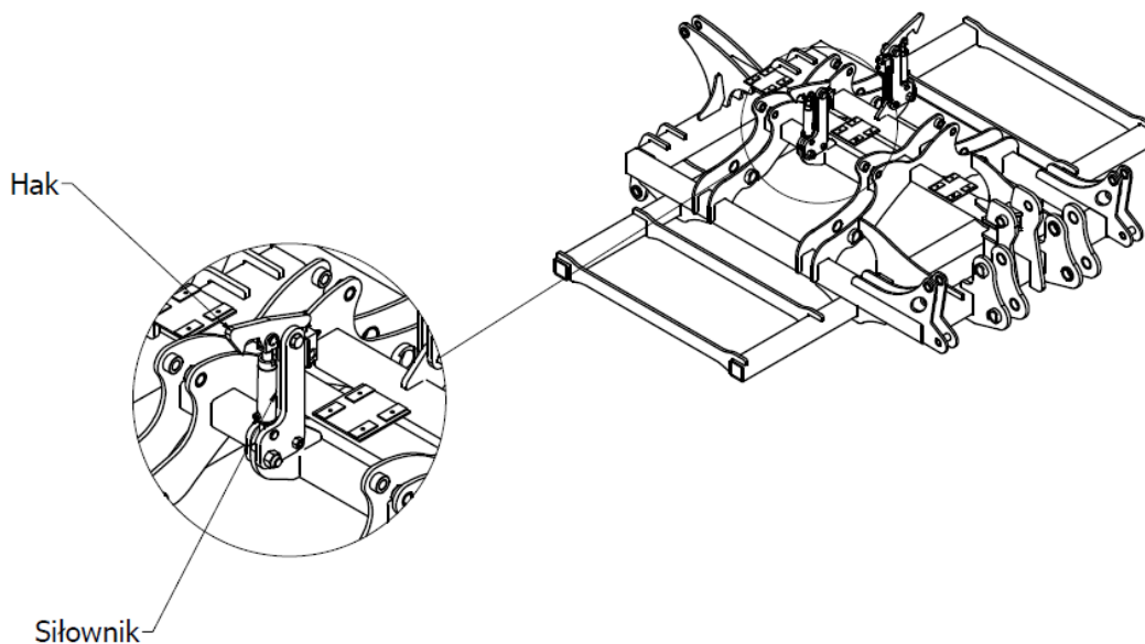
Rys. 4 Rama główna z mechanizmem automatycznej blokady skrzydeł.
