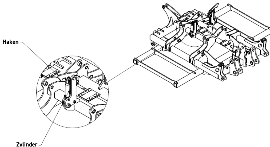
Abb. 4 Hauptrahmen mit automatischer Maschinenflügelverriegelung.
