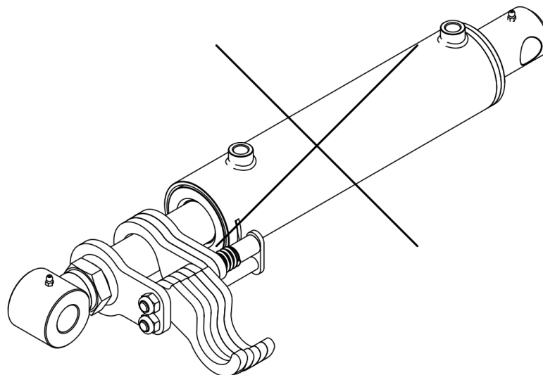
Abb. 12 Inkorrekte Montage der Sperrklinke auf die Pleuellstange des Zylinders. Wenn die Sperrklinken teilweise aus dem Pleuelllager entfernt werden, werden die auf die Pleuellstange wirkenden Kräfte nicht gleichmäßig verteilt und können zum Ausknicken der Pleuellstange führen, was eine Beschädigung der gesamten Pleuellbaugruppe zur Folge hat. Eine solche Einstellung ist unzulässig!
