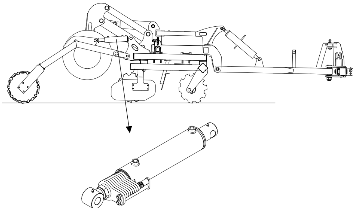
Abb. 10 Zylinder mit an der Kolbenstange befestigten Sperrklinken zur Einstellung der Arbeitstiefe.
