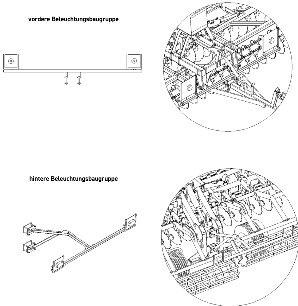
Abb. 13 Vordere und hintere Beleuchtungsbaugruppen und ihre Anordnung.
