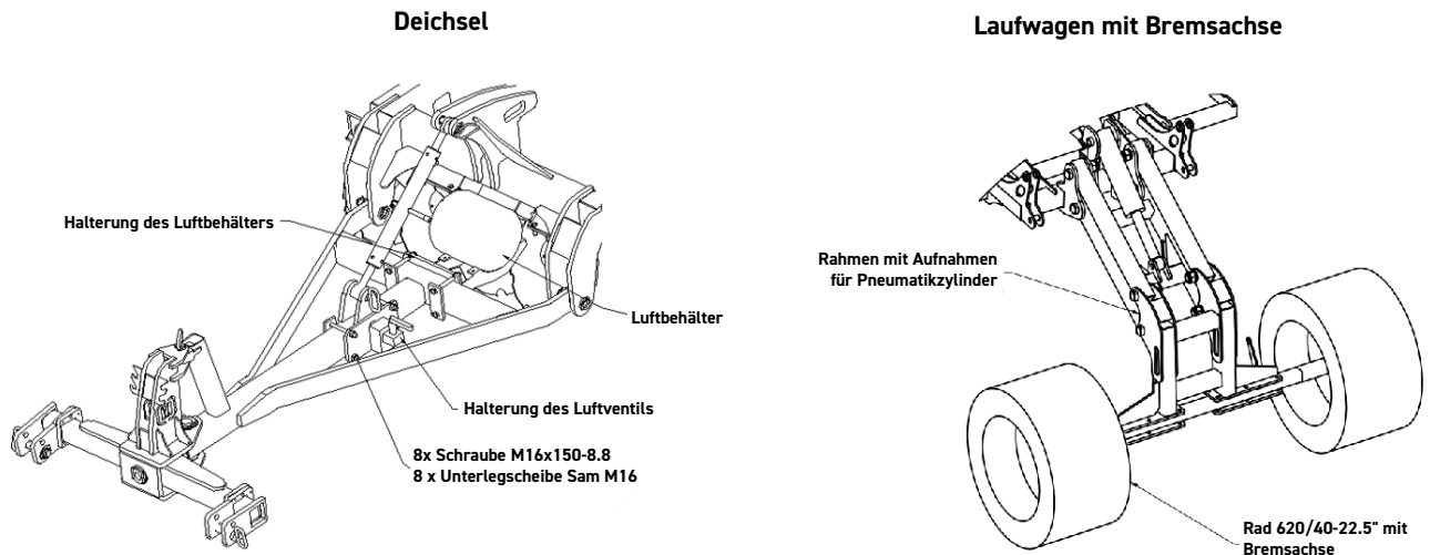
Abb. 14 Pneumatische Anlage der Bremsachse
