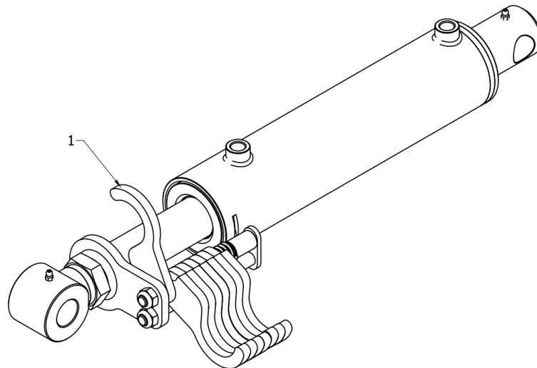
Abb. 11 Korrekte Montage der ersten (1) Sperrklinke auf die Pleuellstange des Zylinders zur Einstellung der Arbeitstiefe der Maschine.
