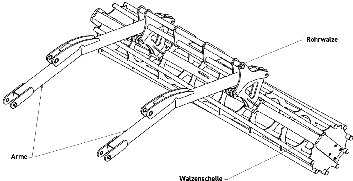
Abb. 2 Verbindung der Arme mit der Walzenschelle.
