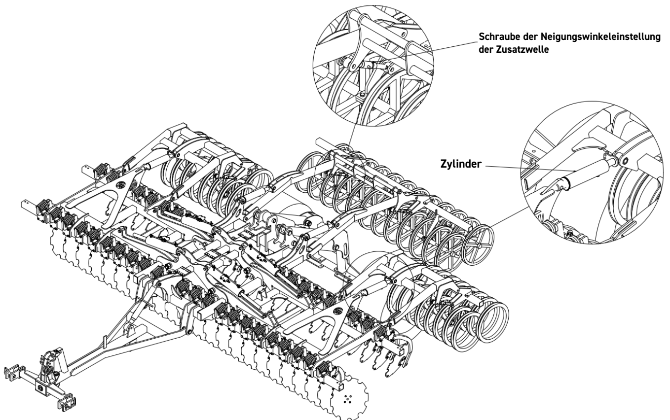
Abb. 9 Hydraulische Tiefeneinstellung der Walze.
