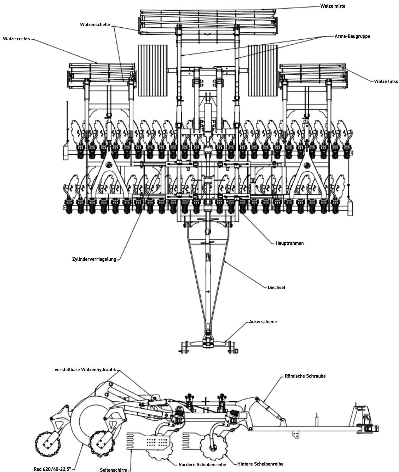
Abb. 1 Scheibenegge SAL-K
