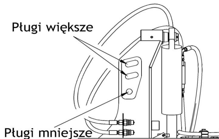
Rys. 7 Zastosowanie odpowiedniego połączenia z łącznikiem górnym pługa.
