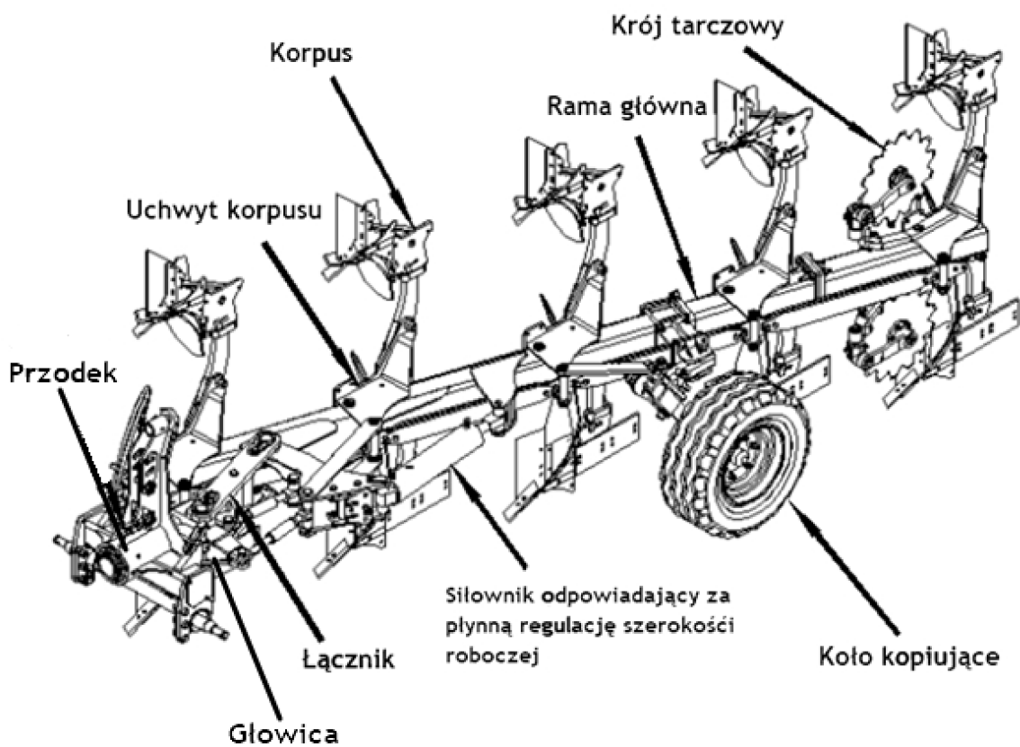
Rys. 2 Budowa pługa ORKAN VARIO.
