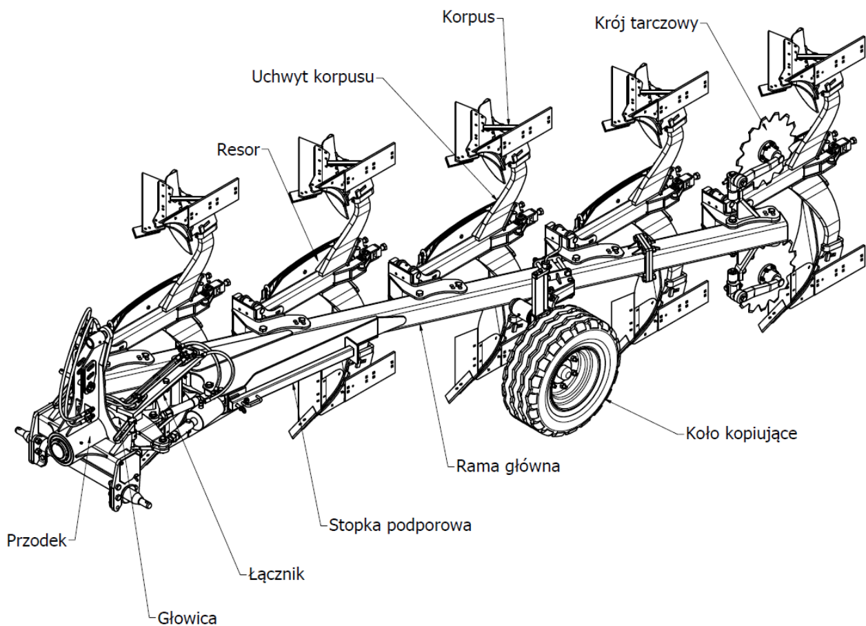
Rys. 3 Budowa pługa ORKAN RESOR oraz narzędzia roboczego.
