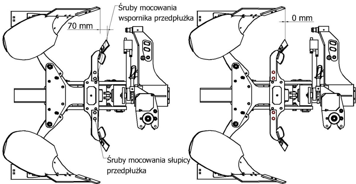
Rys. 14 Schemat mocowania przedpłuźka.
