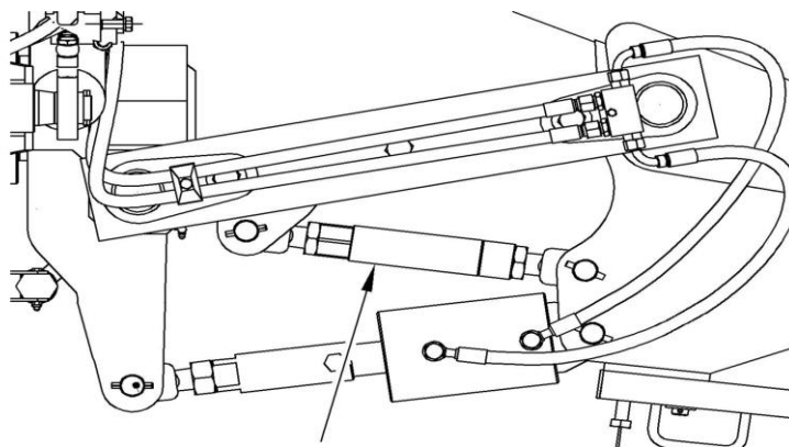
Śruba regulacji pierwszej skiby
