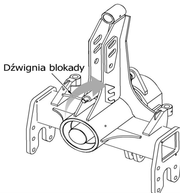
Rys. 5 Schemat dźwigni blokady pługa.
