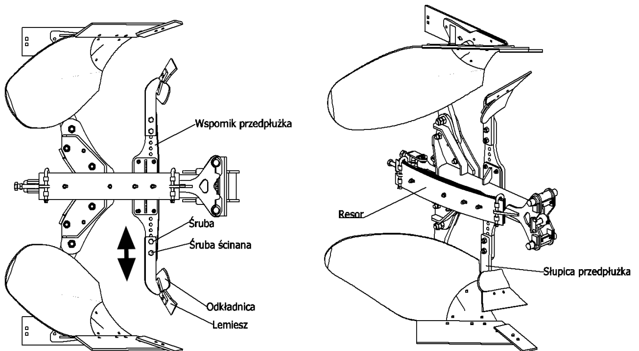
Rys. 15 Budowa przedpłuźka.
