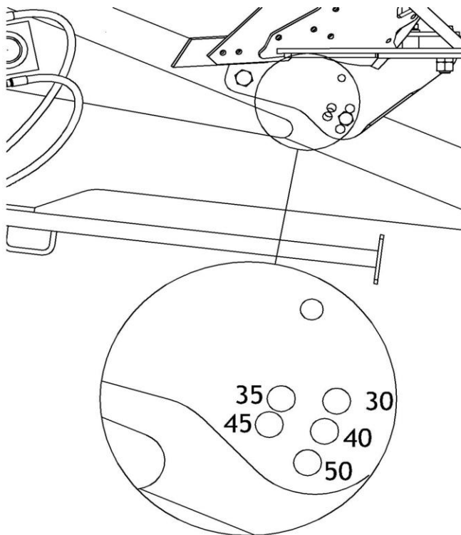
Rys. 9 Otwory regulujące szerokość pracy maszyny.
