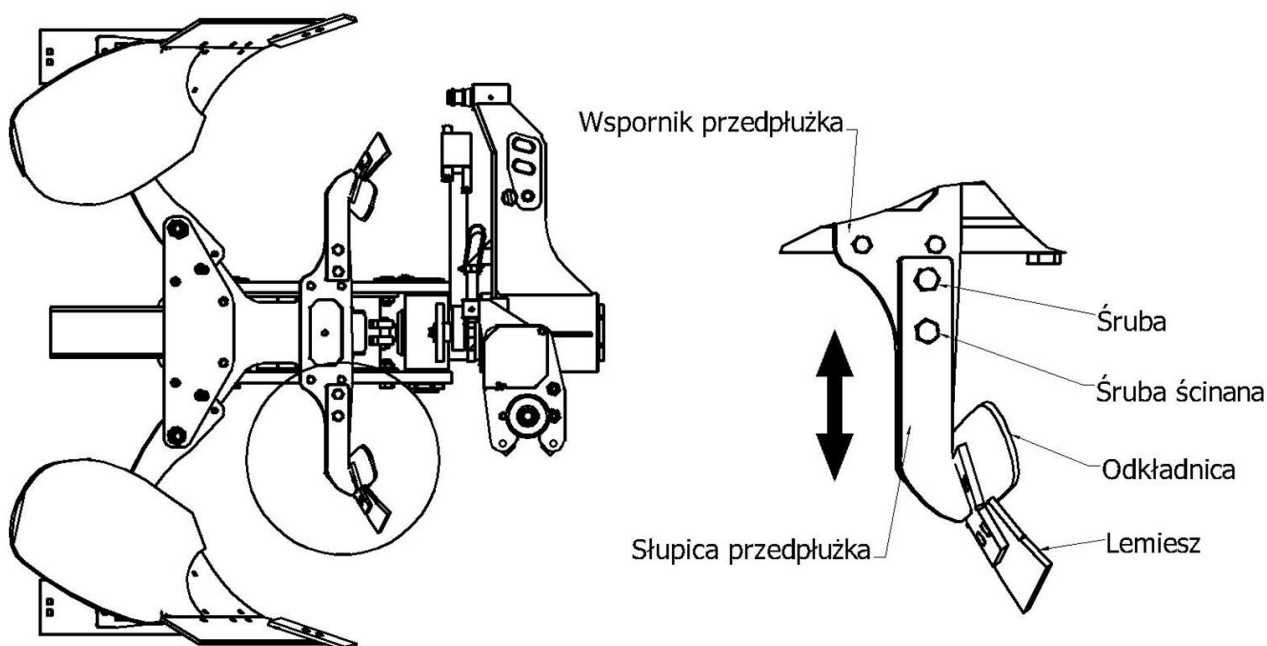
Rys. 13 Budowa przedpłużka.
