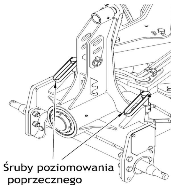
Rys. 12 Śruby służące do poziomowania poprzecznego pługa.
