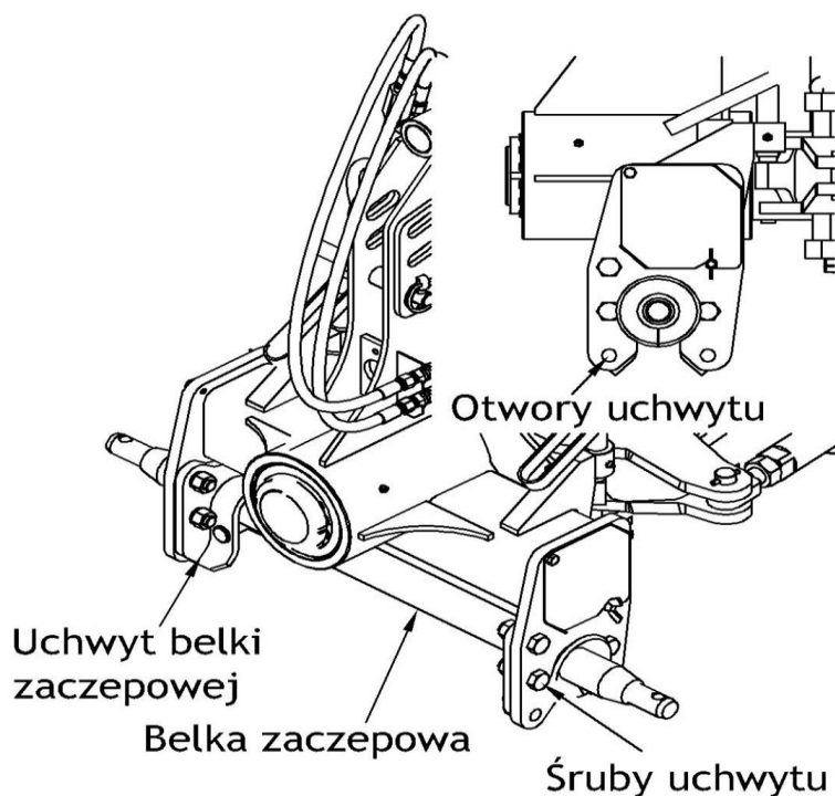
Rys. 8 Schemat regulacji wysokości belki zaczepowej.
