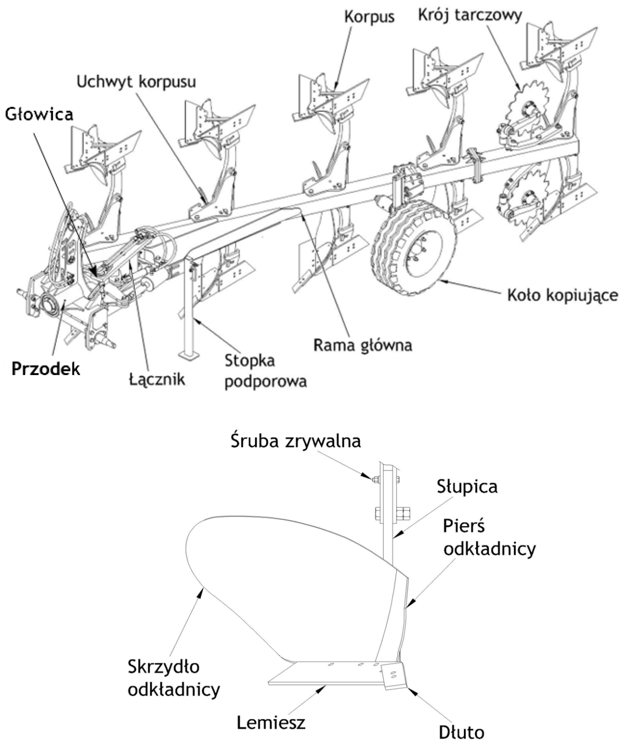
Rys. 1 Budowa pługa ORKAN oraz narzędzia roboczego.
