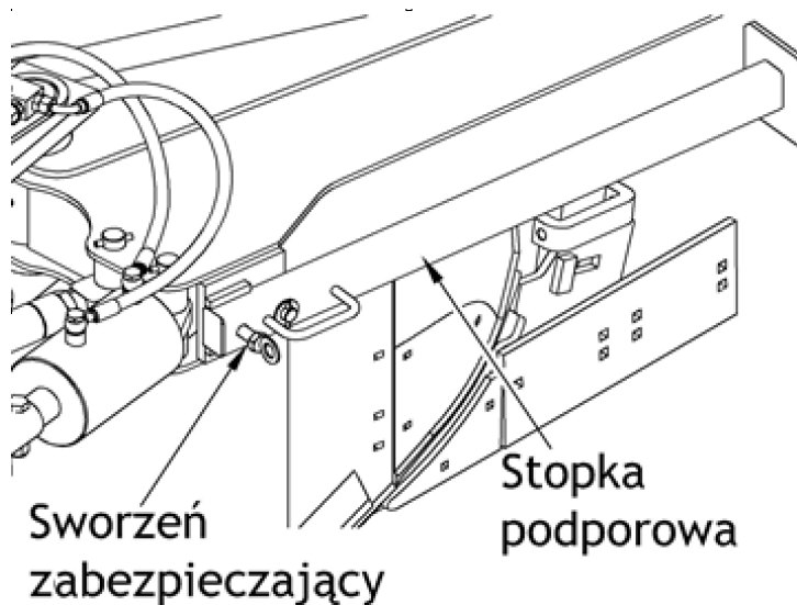
Rys. 6 Stopka podporowa pługa.
