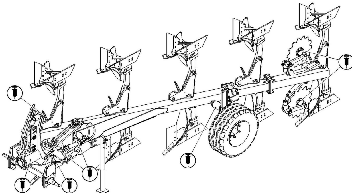
Rys. 13 Punkty smarownicze pługa ORKAN.
