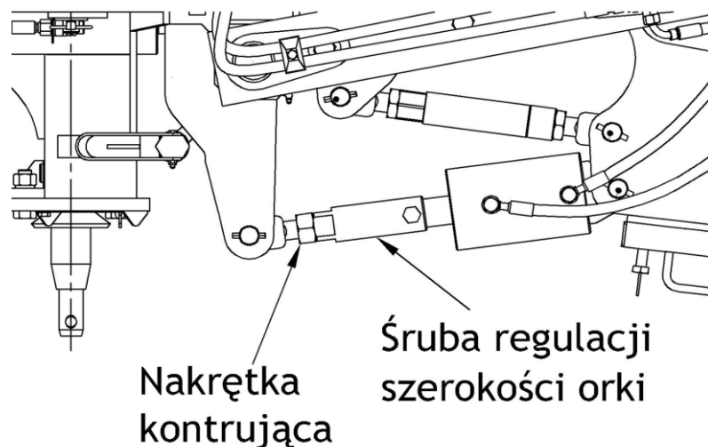
Rys. 10 Regulacja szerokości orki pługa ORKAN.
