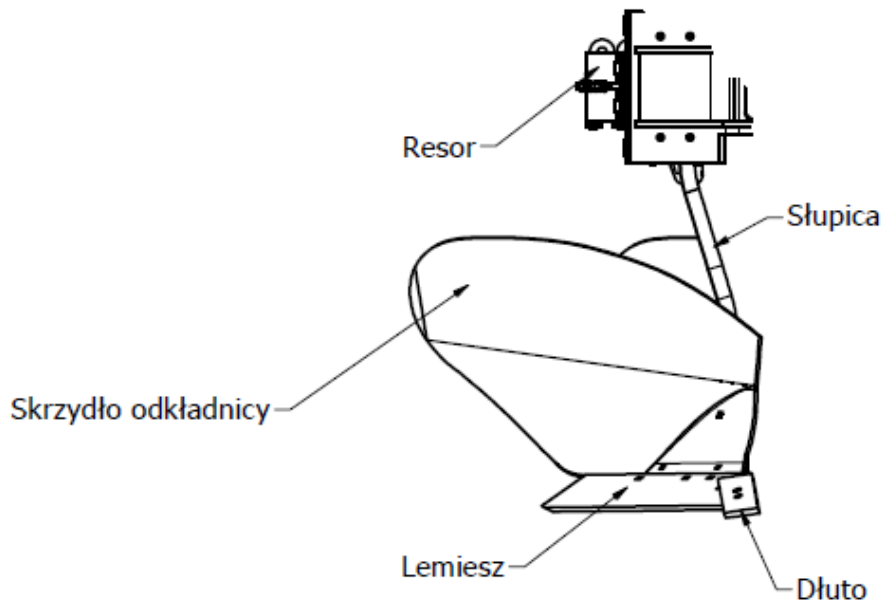
Rys. 4 Budowa narzędzia roboczego ORKAN RESOR.
