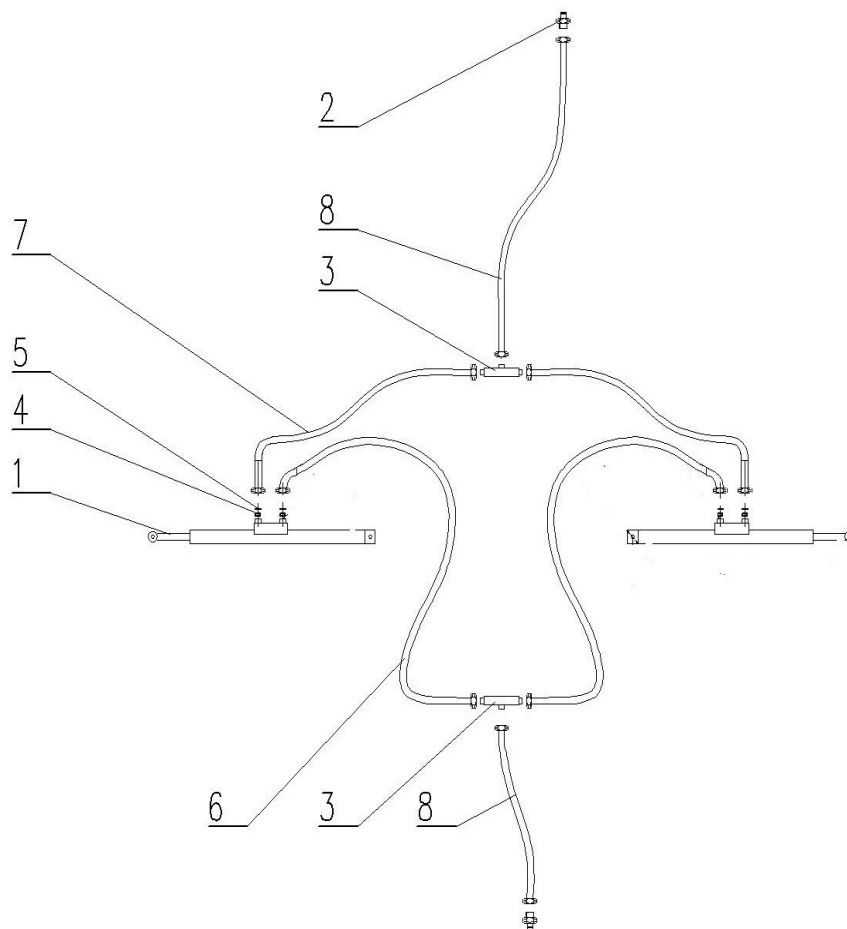
Rys. 8 Schemat układu hydraulicznego wału nożowego 4,0H: 1- siłownik, 2- szybkozłącze, 3- trójnik, 4- kryza, 5- podkładka miedziana, 6,7,8 - przewody hydrauliczne
