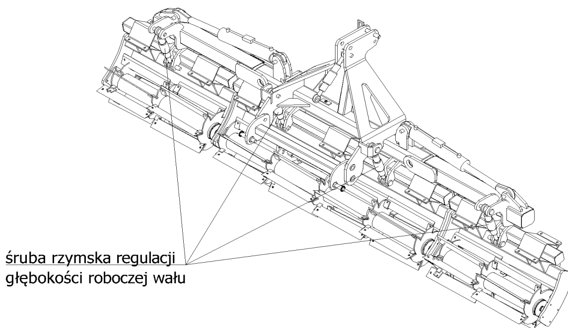
Rys. 7 Regulacja głębokości roboczej wału nożowego
