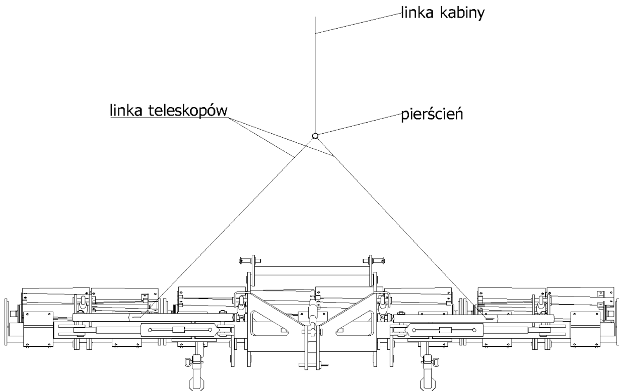
Rys. 5 Sposób mocowania linki zabezpieczenia hydrauliki na wale nożowym 4,0H
