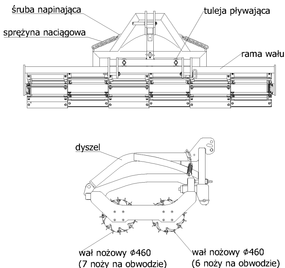
Rys.2 Wał nożowy TANDEM 3,0
